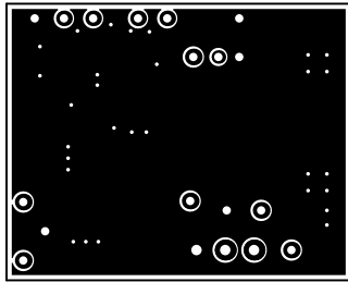
LAYER 3-BOTTOM
