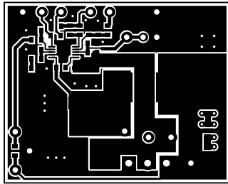
LAYER 1-TOP
