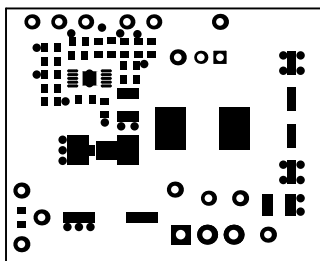
MASK-LAYER 1
