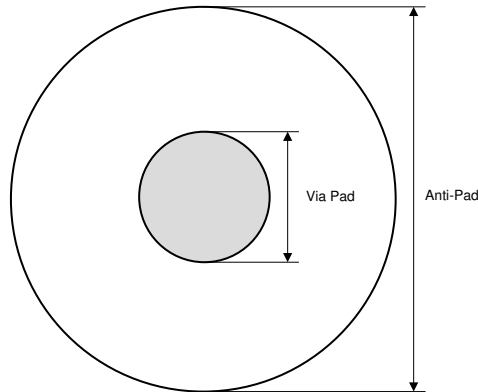
图 3-7. 反焊盘直径
