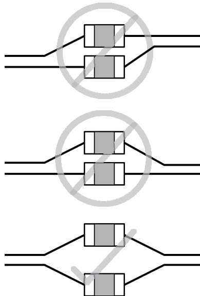
图 3-8. 交流耦合放置
