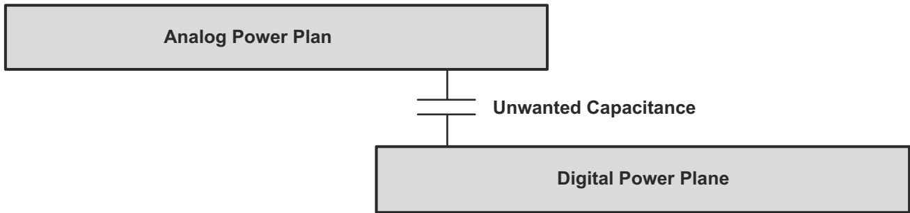
图 2-10. 重叠平面
