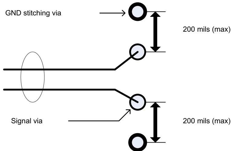
图 2-11. 拼接过孔
