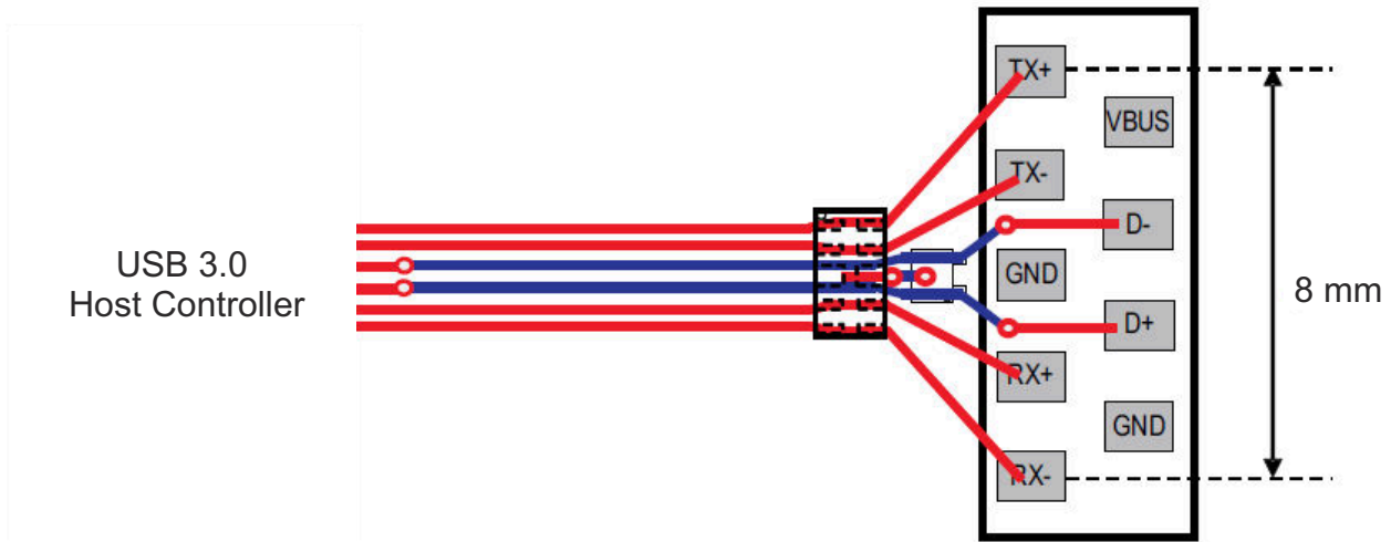
图 3-11. 直通布线
