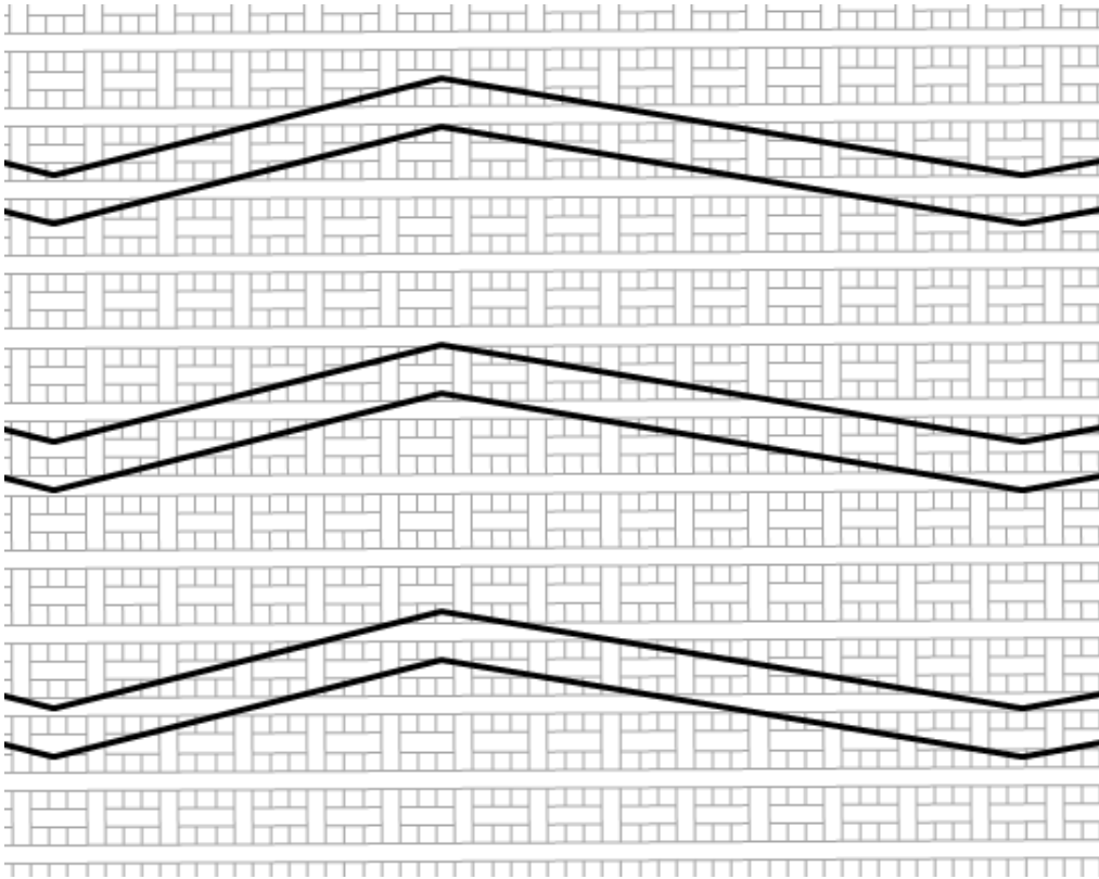
高速差分信号在 PCB 上以锯齿形布线。
