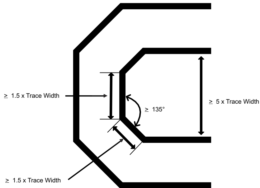
图 3-10. 信号线弯曲规则
