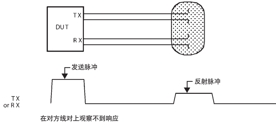
图3. 开路
