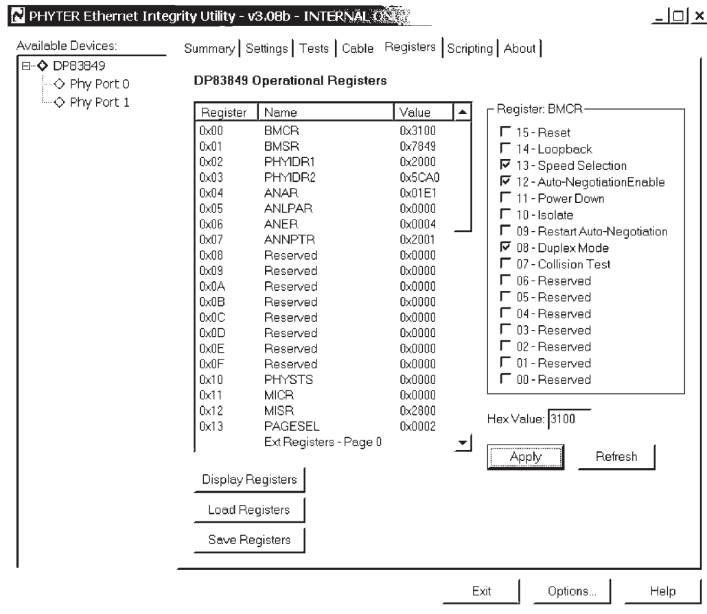
图12. 集成工具 – 寄存器标签
