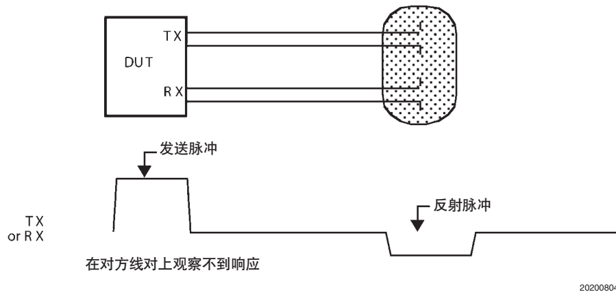
图4. 在单个线对内的短路
