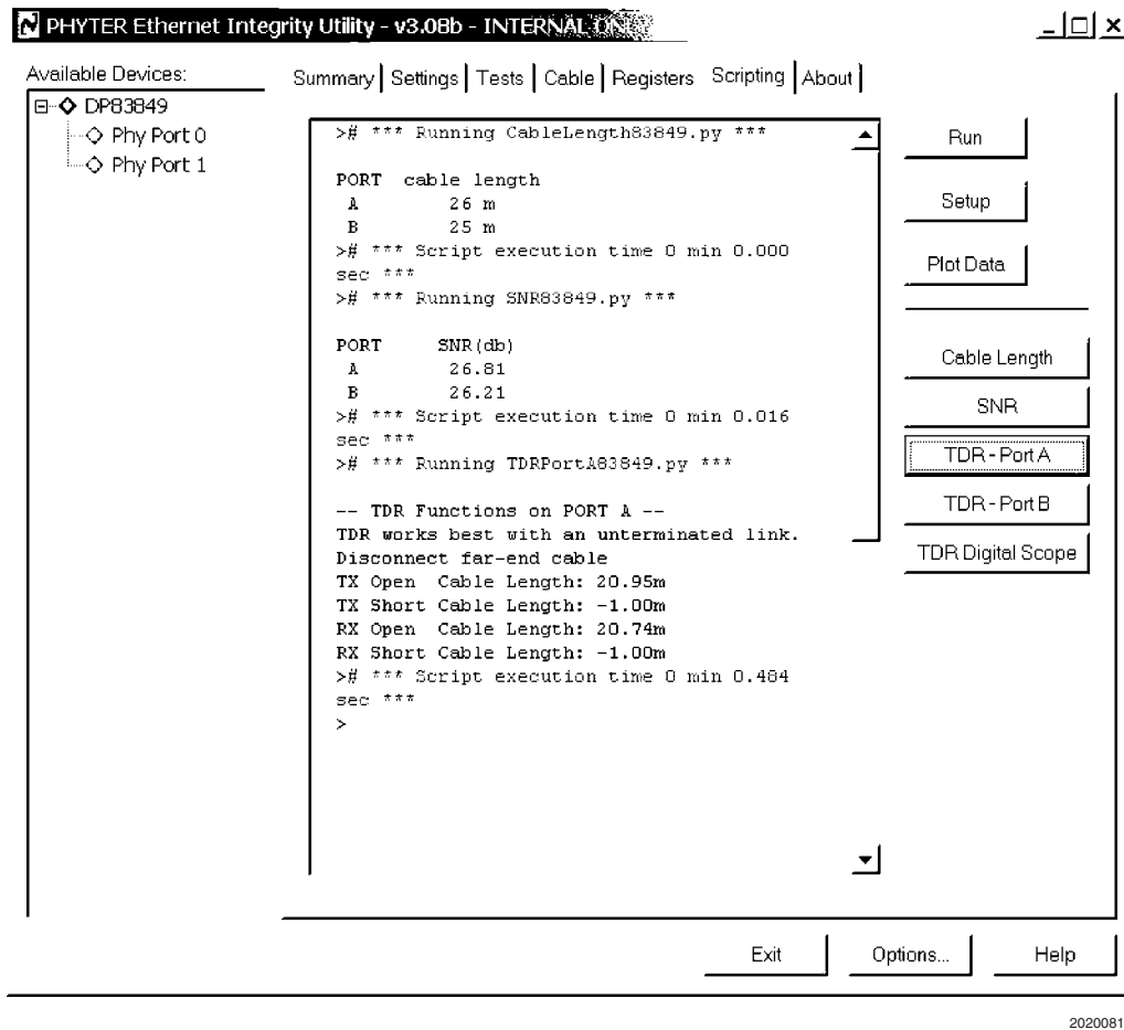
图13. 集成工具 – 脚本标签
