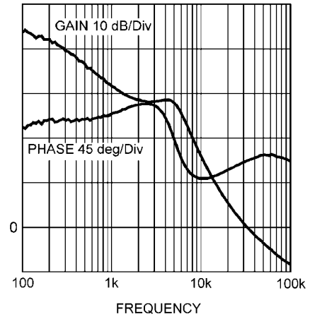
图 5: 总环路增益和相位 ( I_{OUT} = 5 A )
