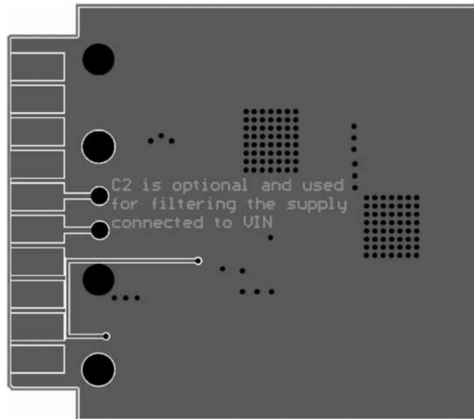
图 7: 底层
