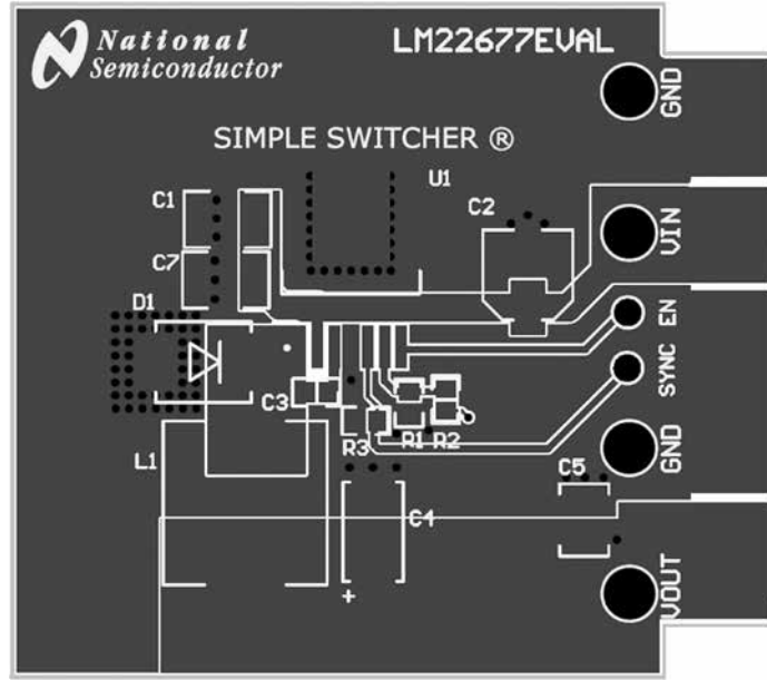
图 6: 顶层
