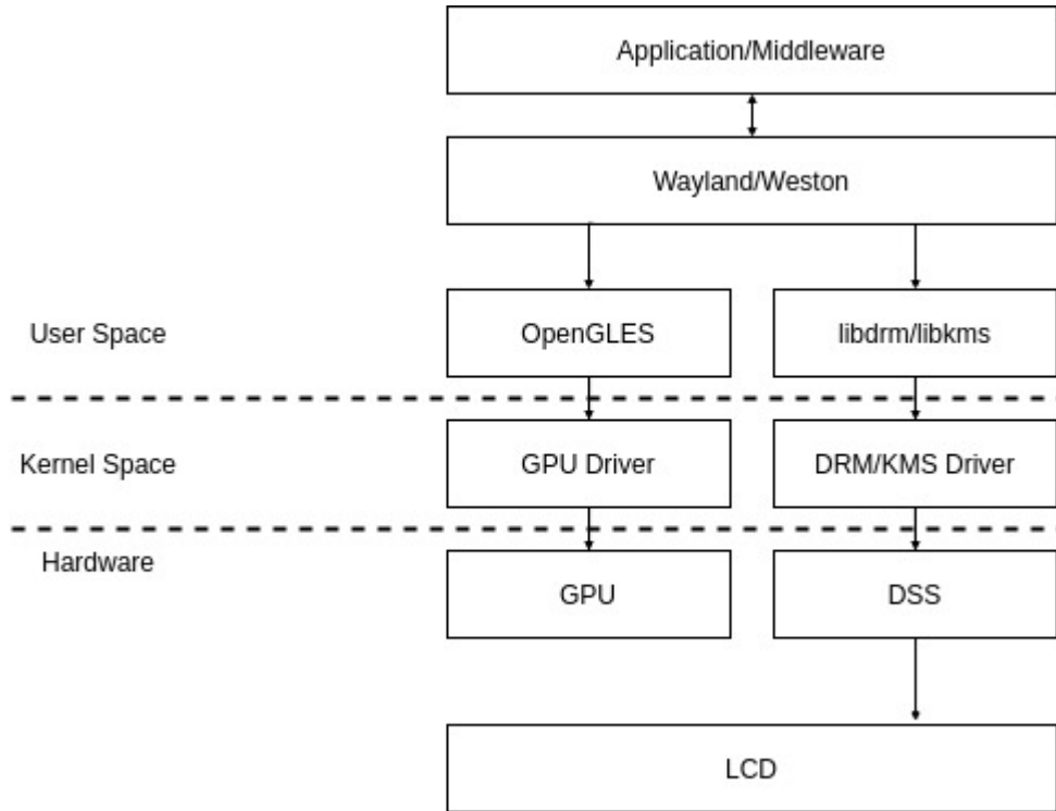
图 2. Linux Weston 系统框架
