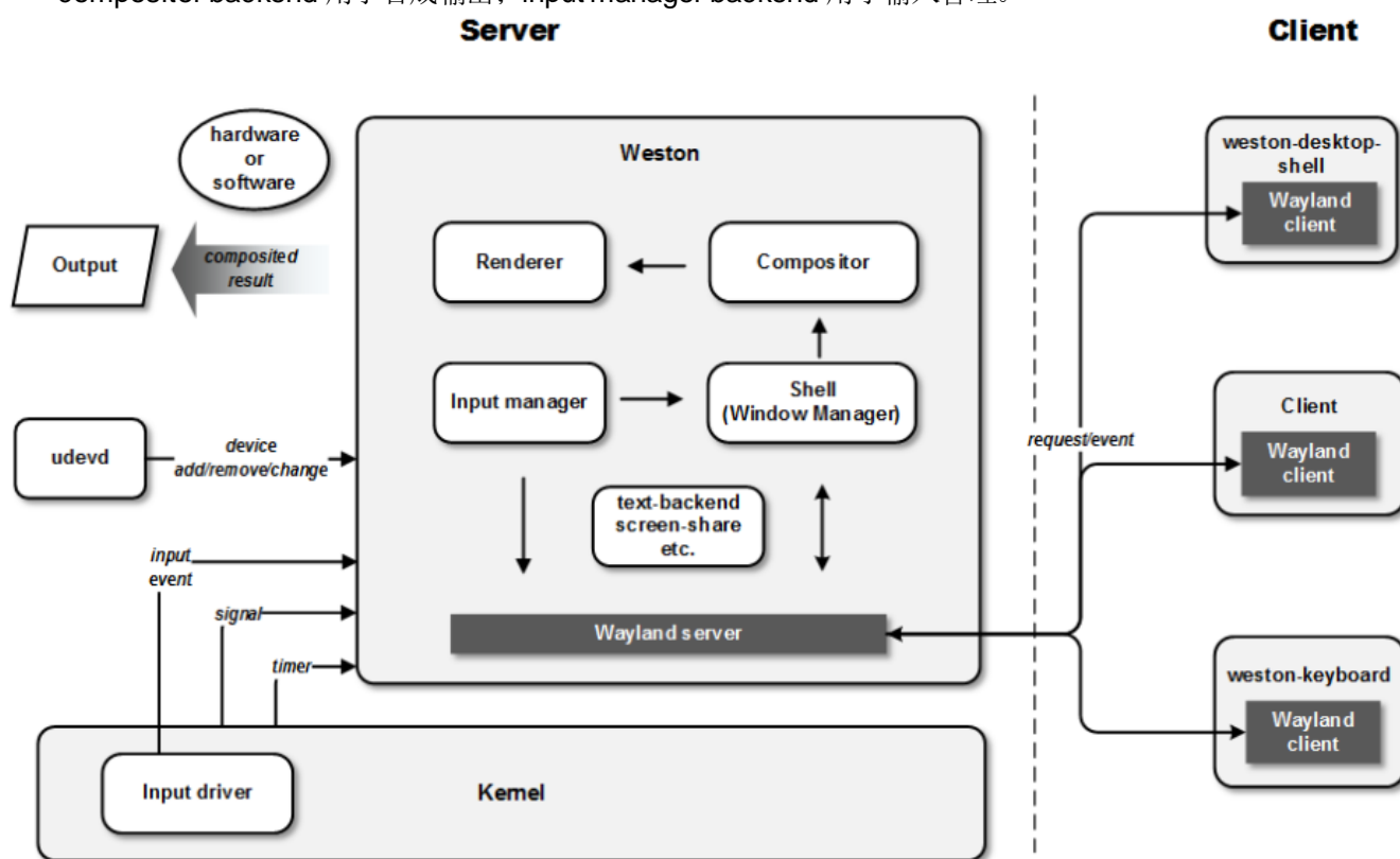
图 1. Weston 框架
