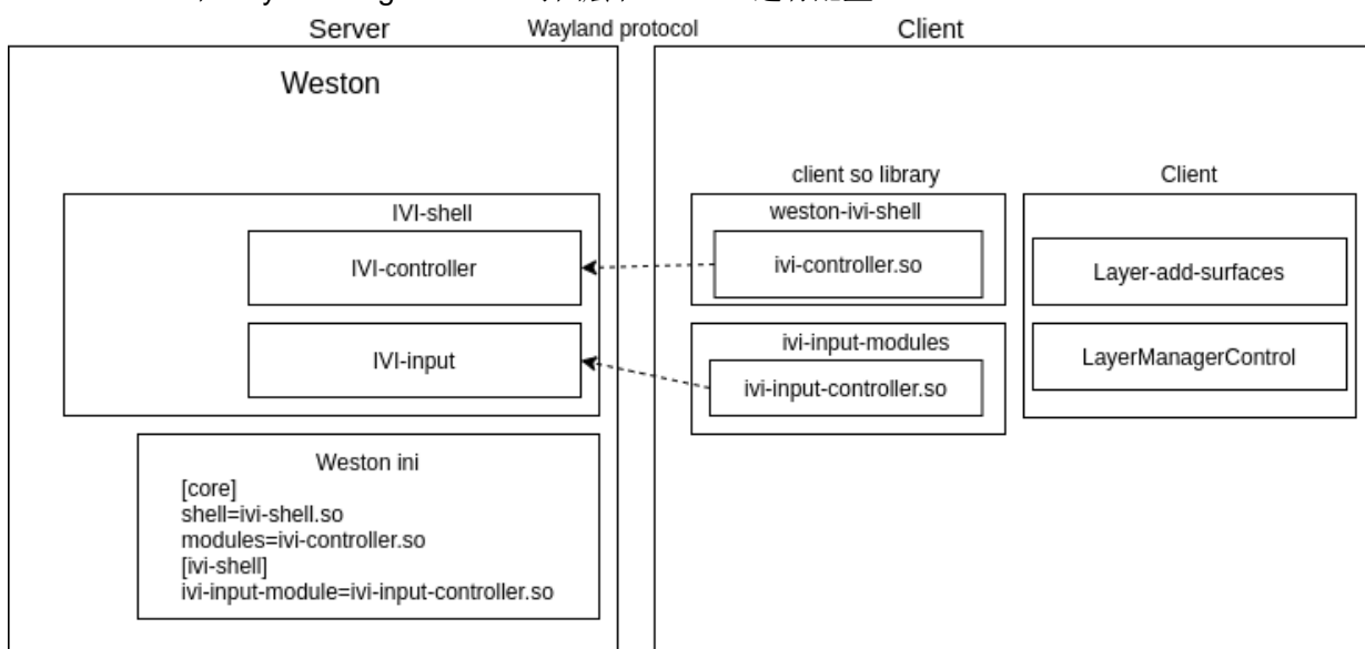
图 3. IVI-shell 框架
