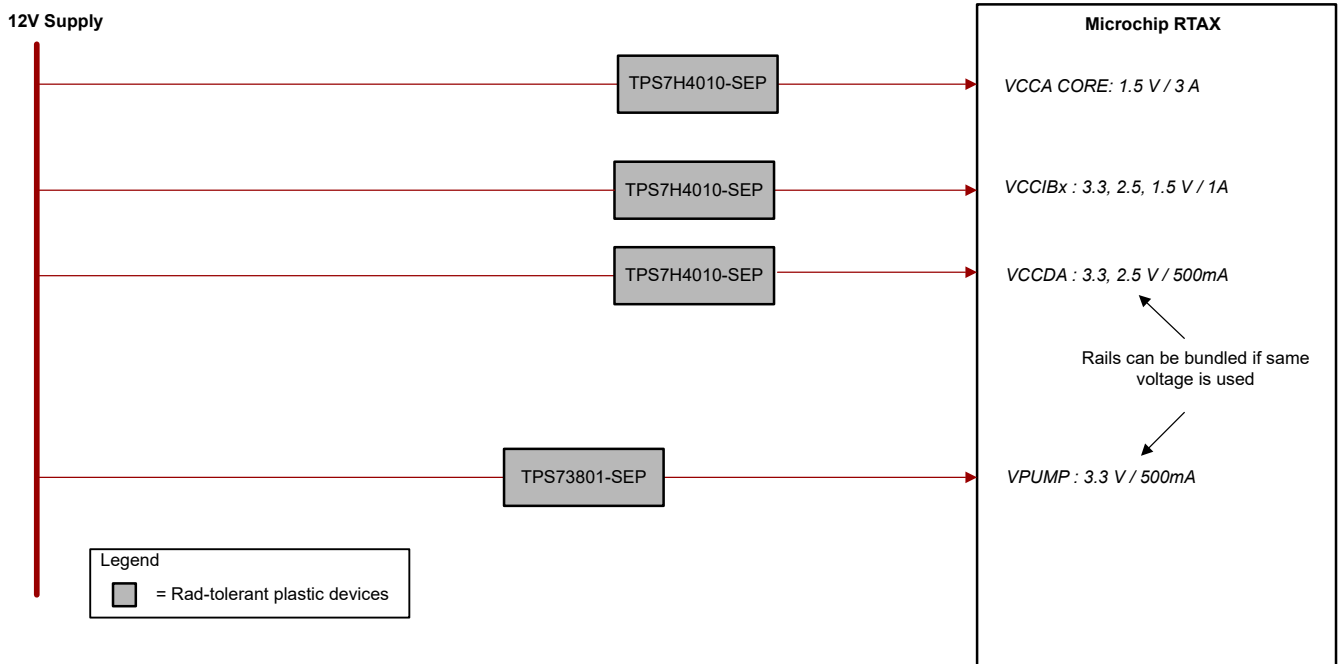
图 4-2. 适用于 RTAX 的耐辐射电源
