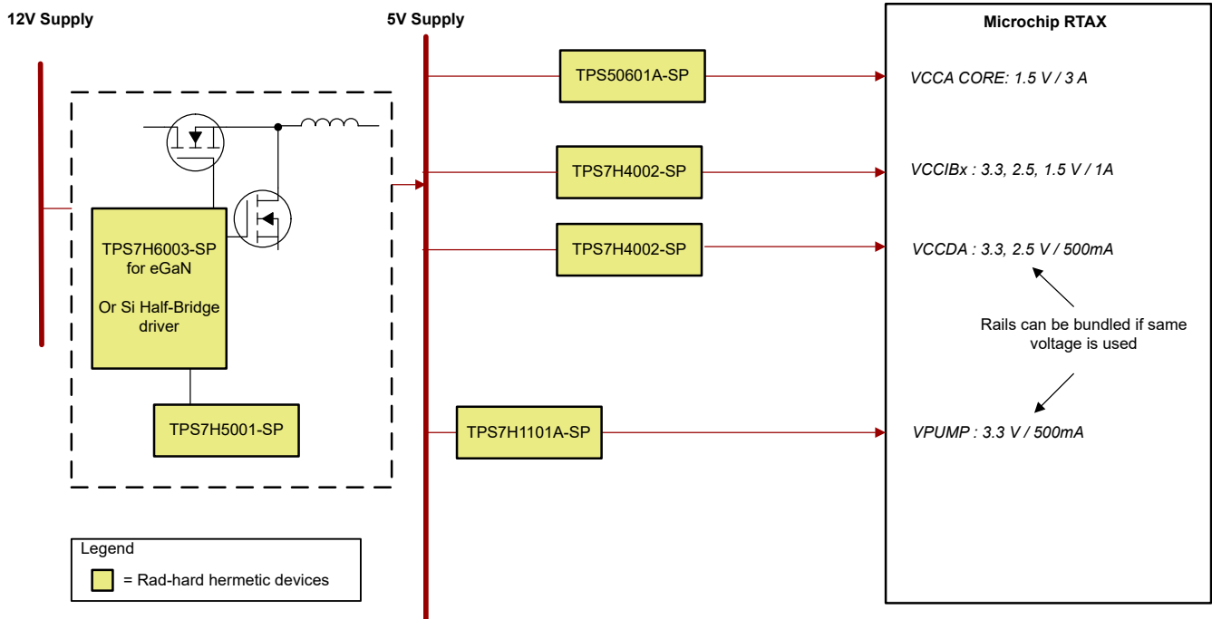
图 4-1. 适用于 RTAX 的耐辐射电源
