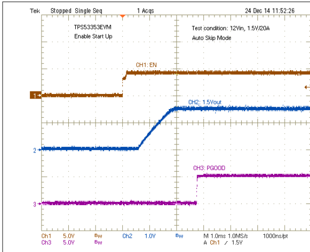
图 8-2. Enable Turnon
