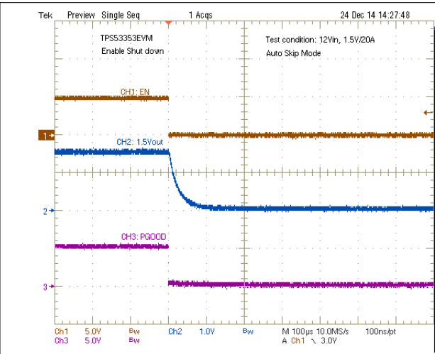
图 8-3. Enable Turnoff
