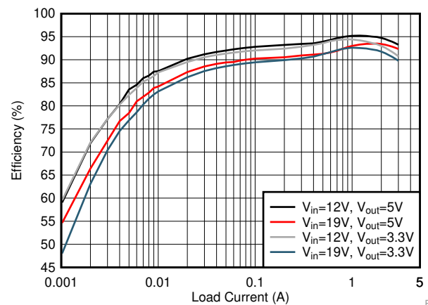
TPS56339 效率
