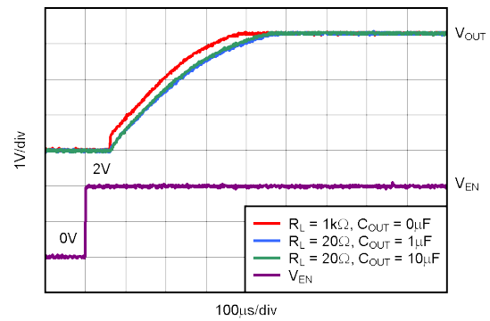
图 5-40. TPS73233 Turn-On Response
