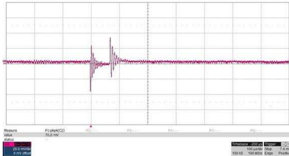
图 7. Ripple Voltage on 3.3-V Load
