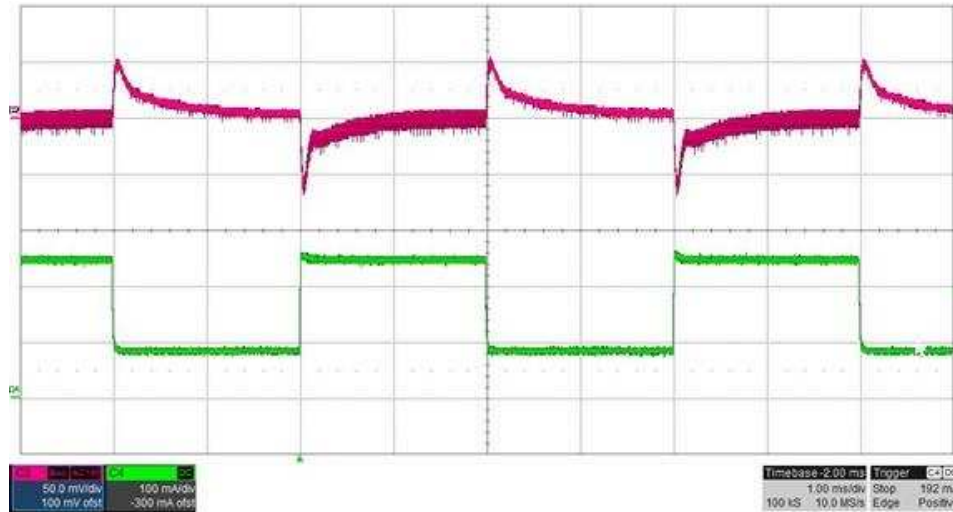
图 8. Load Transients on 5-V Output
