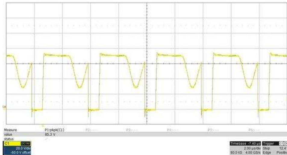
图 9. Switching Waveforms for Q1
