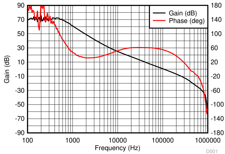
图 3-2. 环路响应测量 ( V_{IN} = 12V , V_{OUT} = 1.2V , I_{OUT} = 3000mA , JP2 打开)
