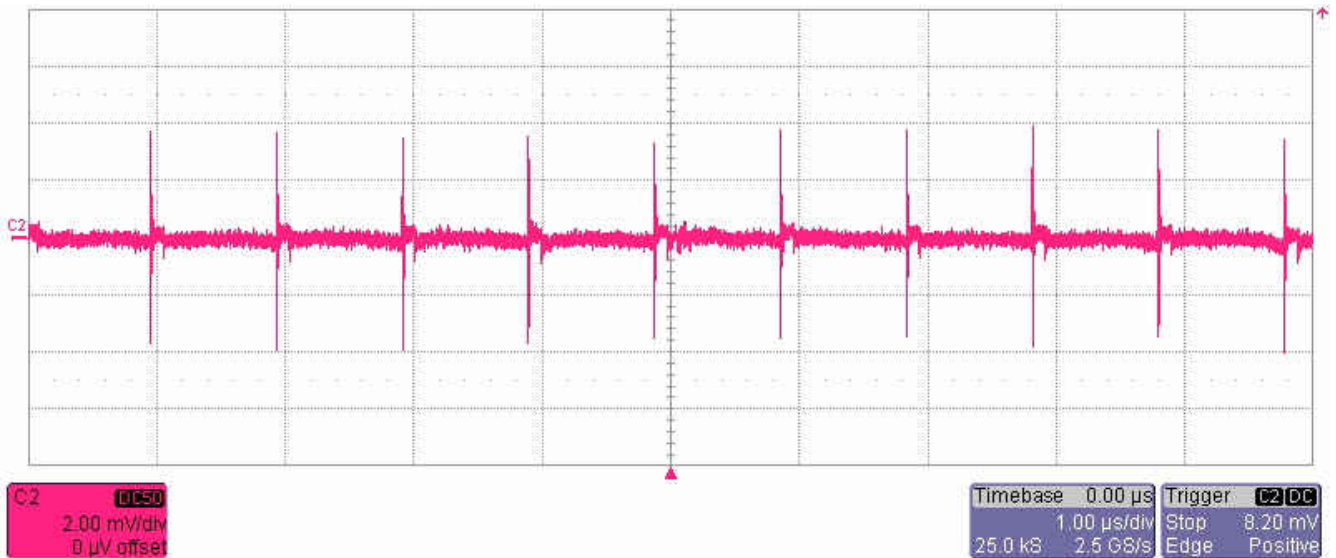
图 A-1. 输出电压纹波, 于 J4 处测量
