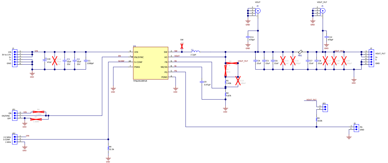
图 5-1. TPS62913EVM-077 原理图
