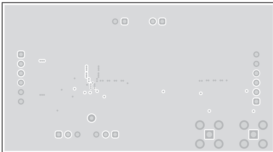
图 4-3. 内层 1
