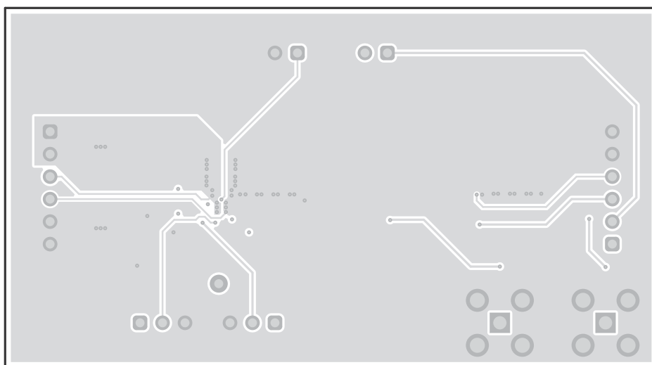
图 4-4. 内层 2
