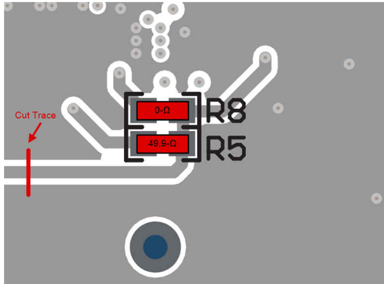
图 1-1. 环路响应测量修改 (底层)
