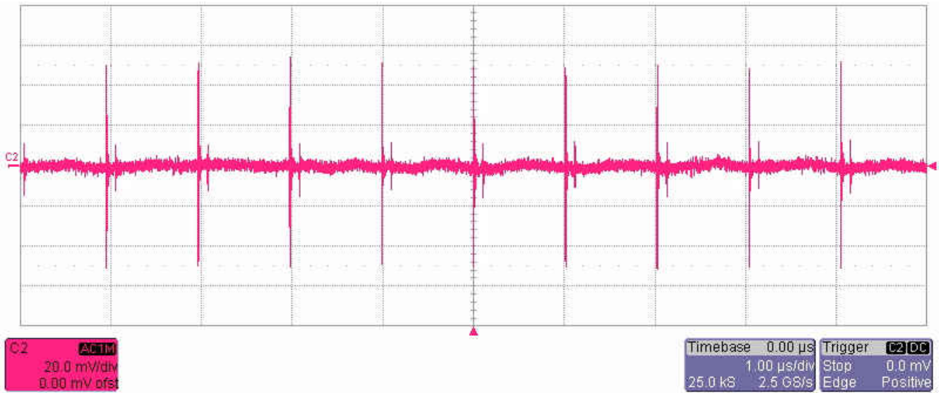
图 2-3. 输出电压纹波, 跨 C4 测量, 使用 10x 探头
