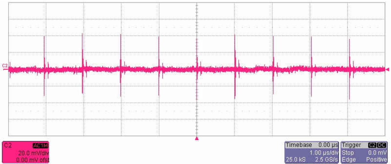
图 2-5. 输出电压纹波, 跨 C7 测量, 使用 1x 探头
