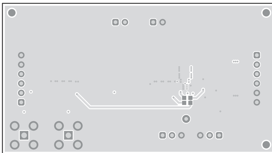
图 4-6. 底层 ( 镜像 )
