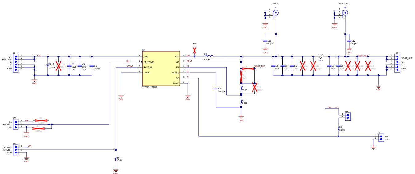
图 5-2. TPS62912EVM-077 原理图
