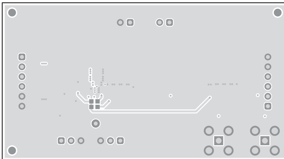
图 4-5. 底层
