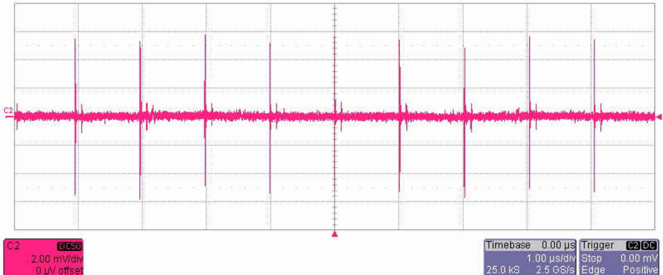
图 2-1. 输出电压纹波, 于 J4 处测量
