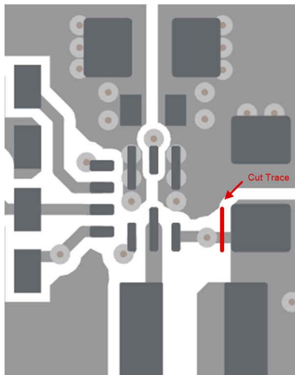
图 1-2. 环路响应测量修改 (顶层)
