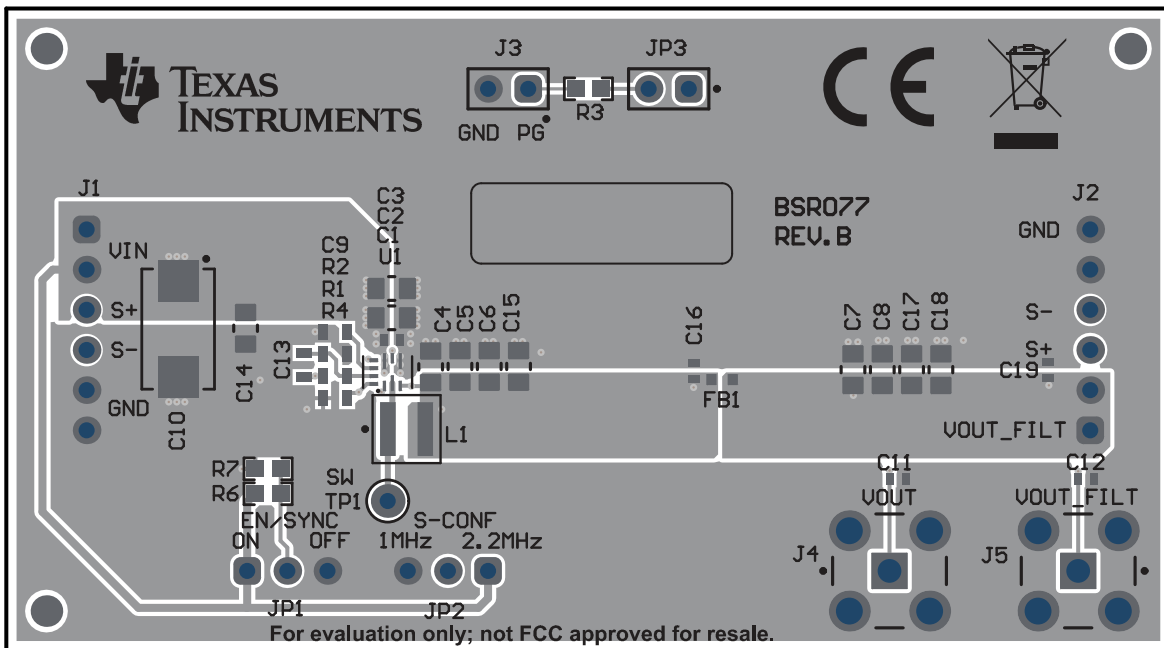
图 4-1. 顶层装配图
