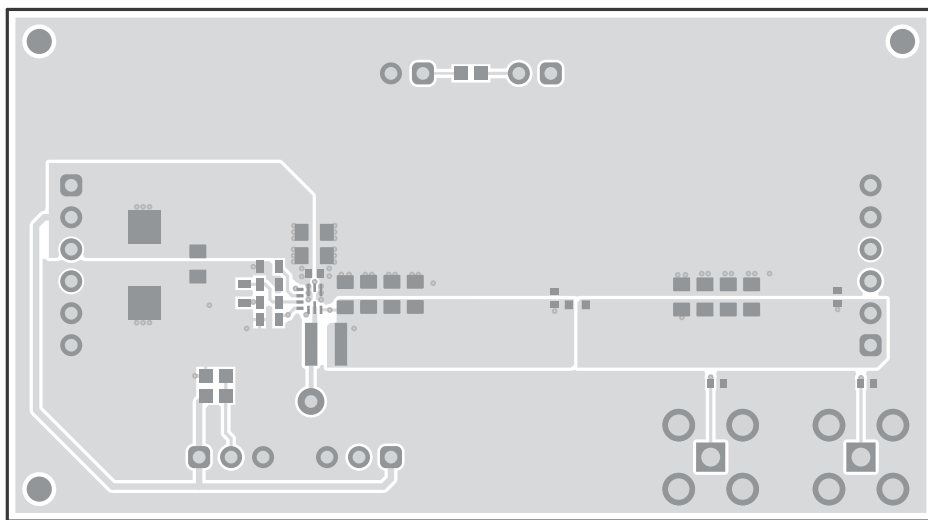
图 4-2. 顶层
