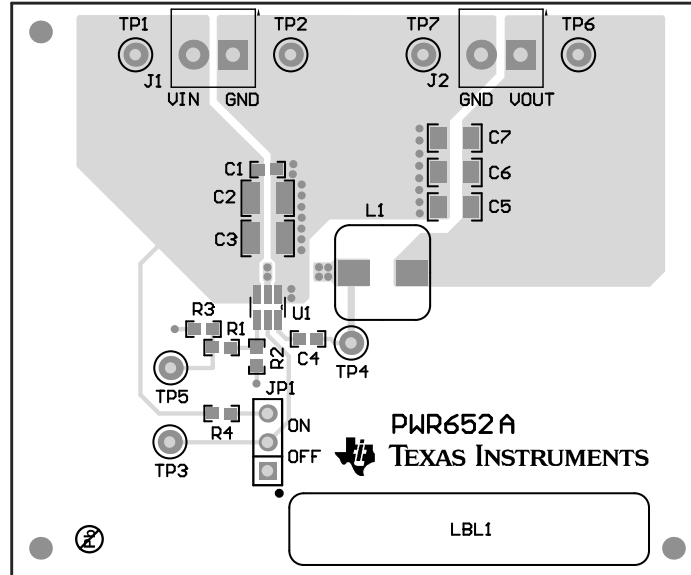
图 5-1. 顶层装配图
