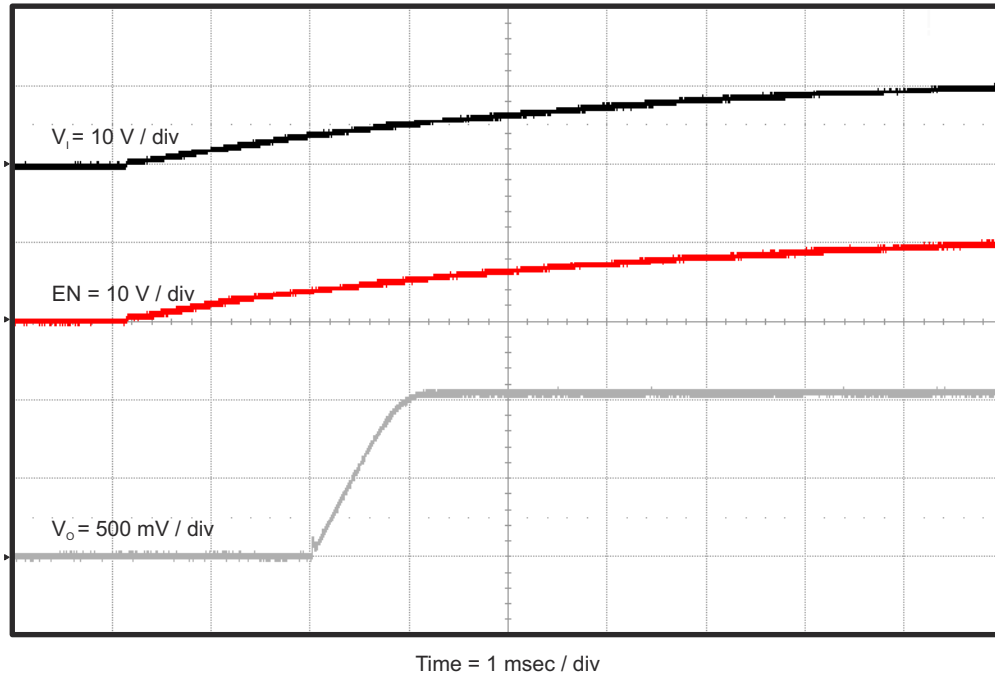
图 4-11. TPS563200EVM-652 相对于 V_{IN} 的启动
