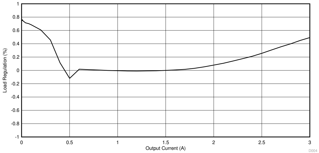
图 4-4. TPS563200EVM-652 负载调整，12V 输入
