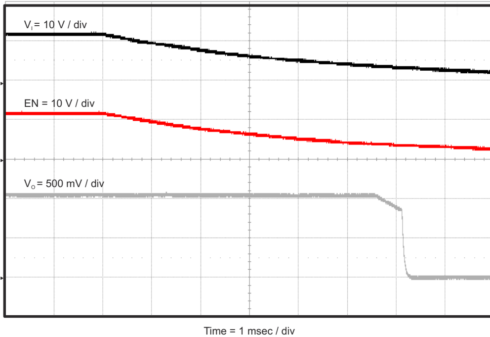
图 4-13. TPS563200EVM-652 相对于 V_{IN} 的关断
