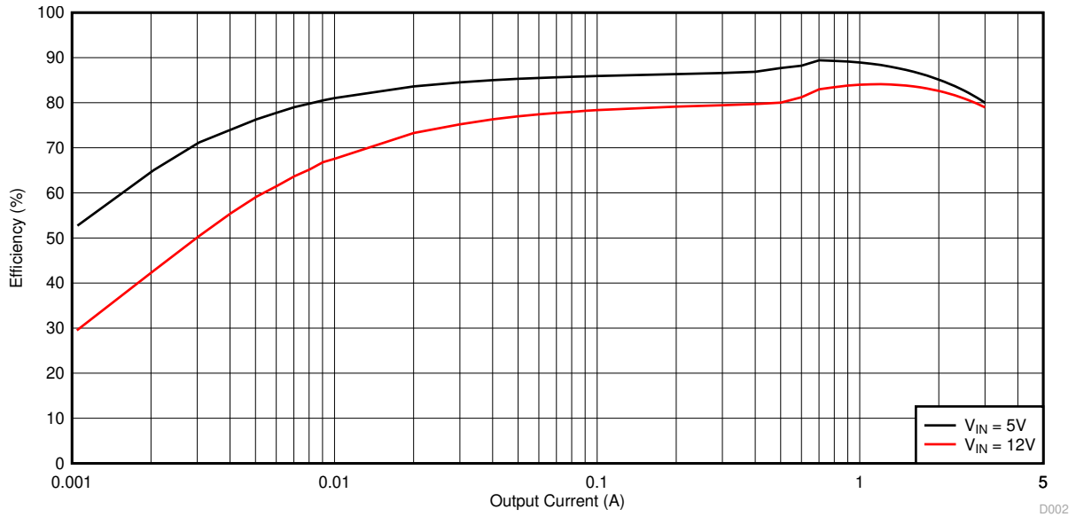
图 4-2. TPS563200EVM-652 轻负载效率
