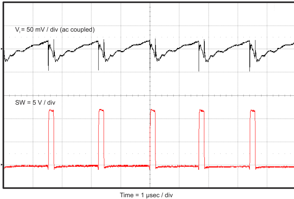
图 4-10. TPS563200EVM-652 输入电压纹波， I_{OUT} = 3\text{A}
