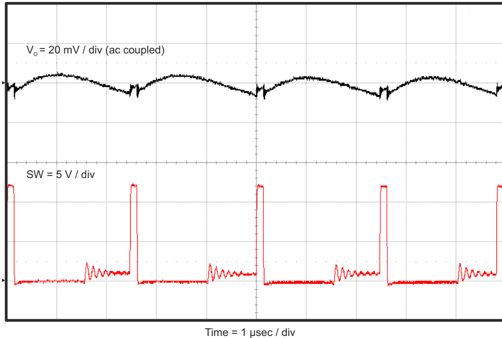
图 4-8. TPS563200EVM-652 输出电压纹波， I_{OUT} = 300\text{mA}
