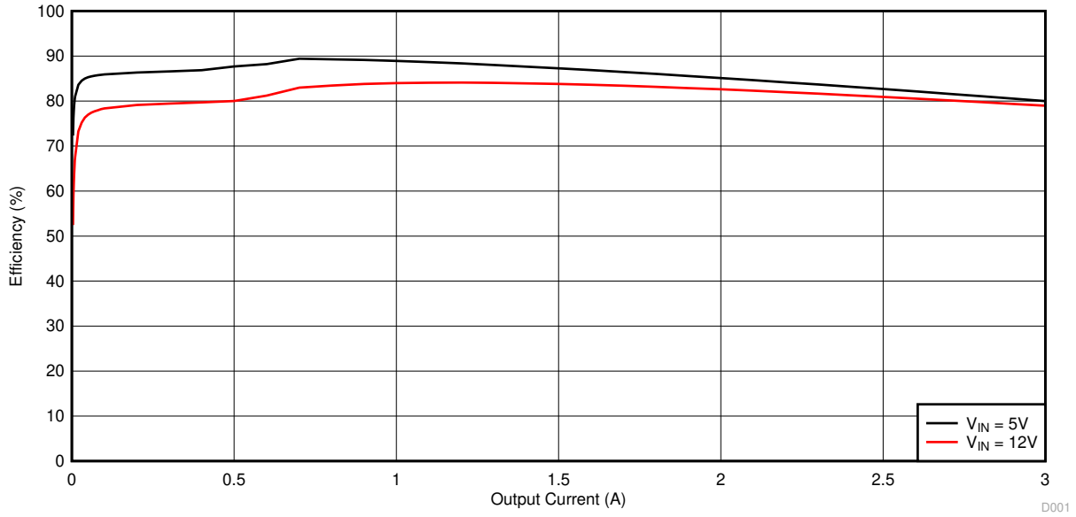
图 4-1. TPS563200EVM-652 效率
