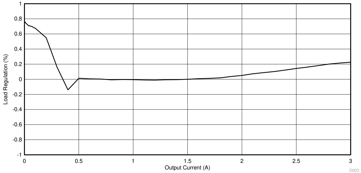
图 4-3. TPS563200EVM-652 负载调整，5V 输入
