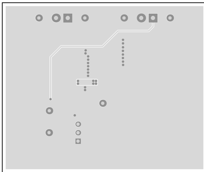
图 5-3. 底层
