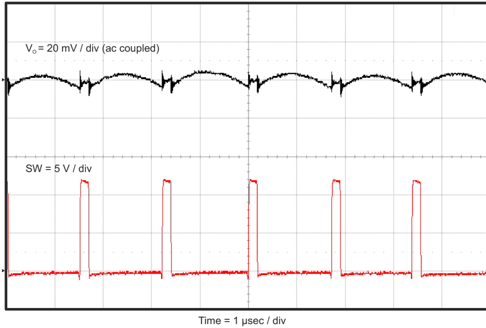
图 4-7. TPS563200EVM-652 输出电压纹波， I_{OUT} = 3\text{A}
