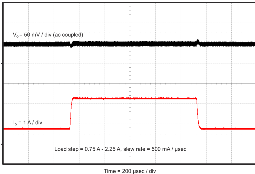
图 4-6. TPS563200EVM-652 负载瞬态响应，25% 至 75% 负载阶跃
