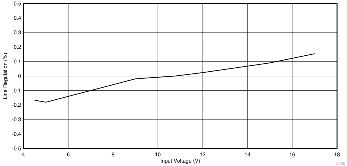
图 4-5. TPS563200EVM-652 线性调整率
