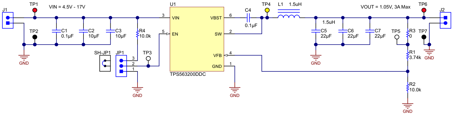
图 6-1. TPS563200EVM-652 原理图
