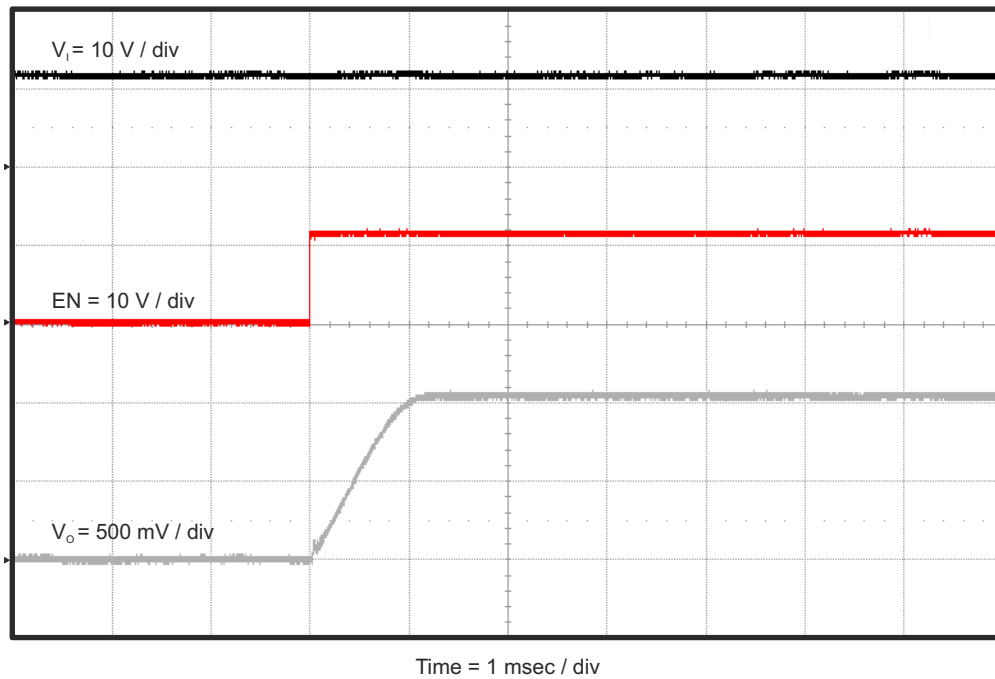
图 4-12. TPS563200EVM-652 相对于 EN 的启动
