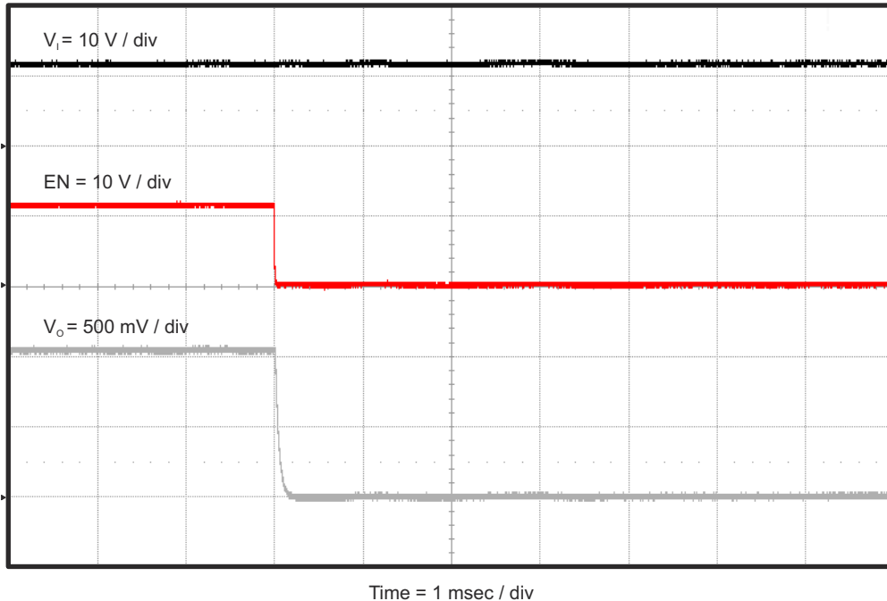
图 4-14. TPS563200EVM-652 相对于 EN 的关断
