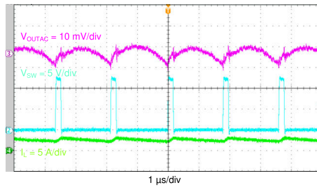
图 4-7. 输出电压纹波, I_{OUT} = 2.5\text{ A}
