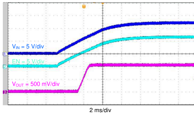
图 4-10. 相对于 V_{IN} 的启动
