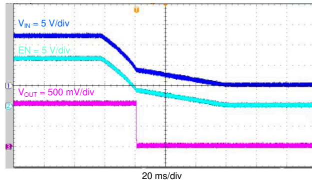
图 4-12. 相对于 V_{IN} 的关断
