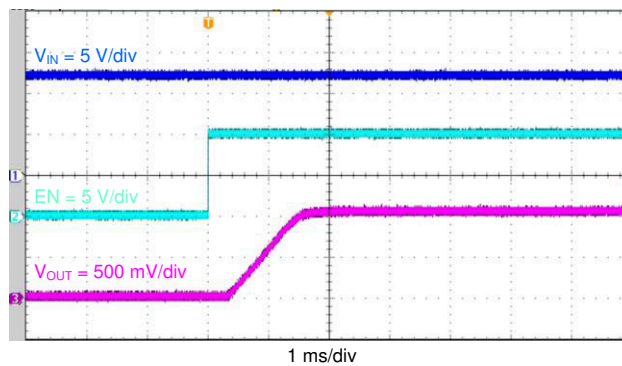
图 4-11. 相对于 EN 的启动
