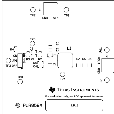
图 5-1. 顶层装配图
