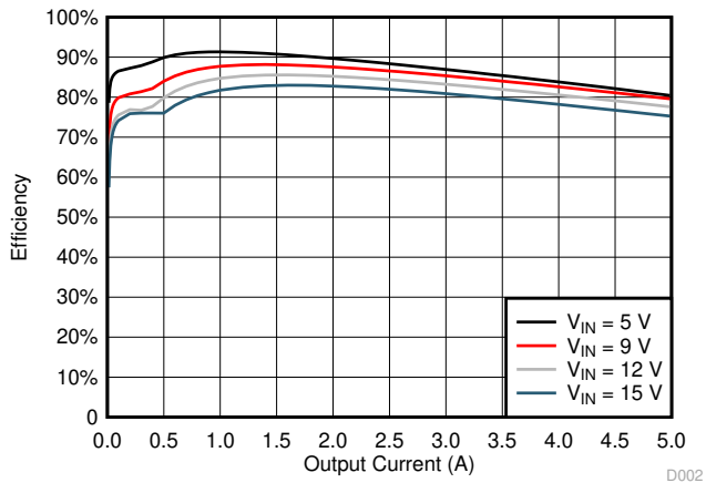
图 4-2. 轻负载效率
