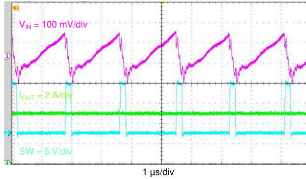
图 4-9. 输入电压纹波
