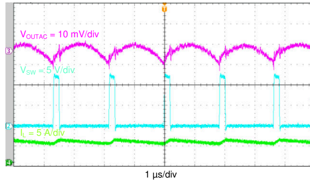
图 4-6. 输出电压纹波, I_{OUT} = 5\text{ A}
