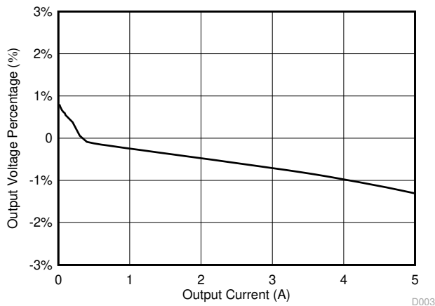
图 4-3. 负载调整率
