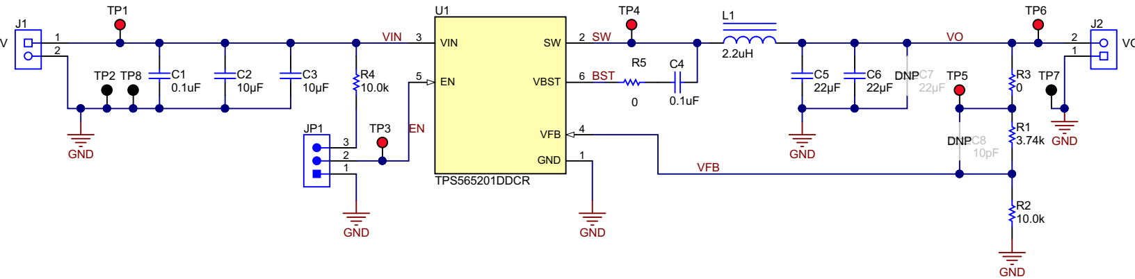
图 6-1. TPS565201EVM-858 原理图
