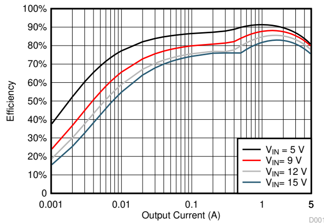
图 4-1. 效率
