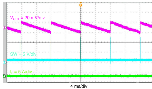
图 4-8. TPS565201 输出电压纹波, 无负载
