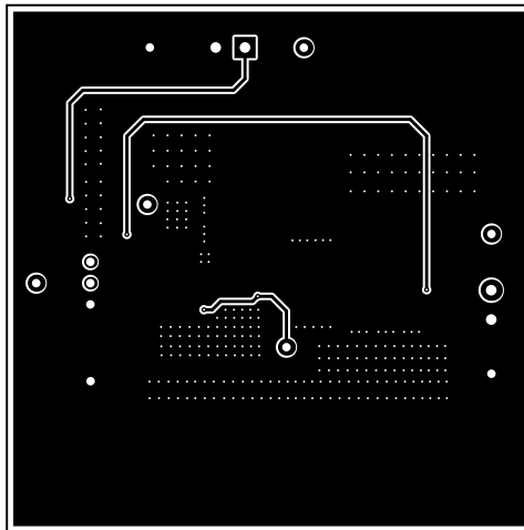
图 5-2. 顶层
