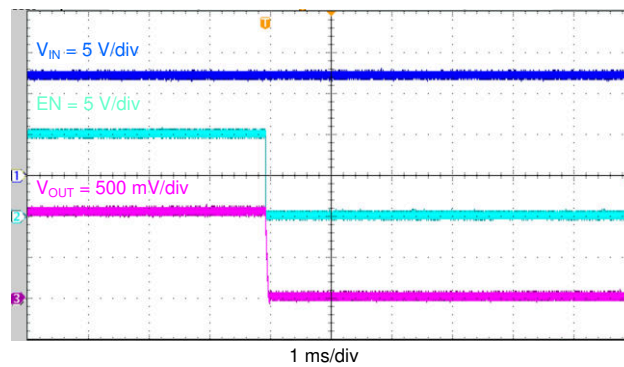
图 4-13. 相对于 EN 的关断
