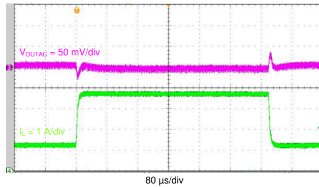
图 4-5. 负载瞬态响应，1.25A 至 3.75A
