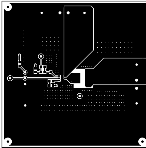
图 5-3. 底层
