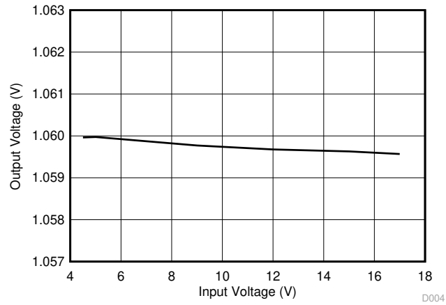
图 4-4. 线性调整率
