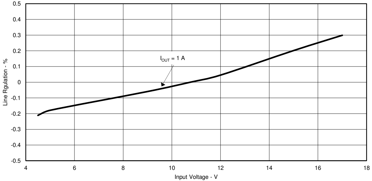
图 4-4. TPS562209EVM-601 线性调整率
