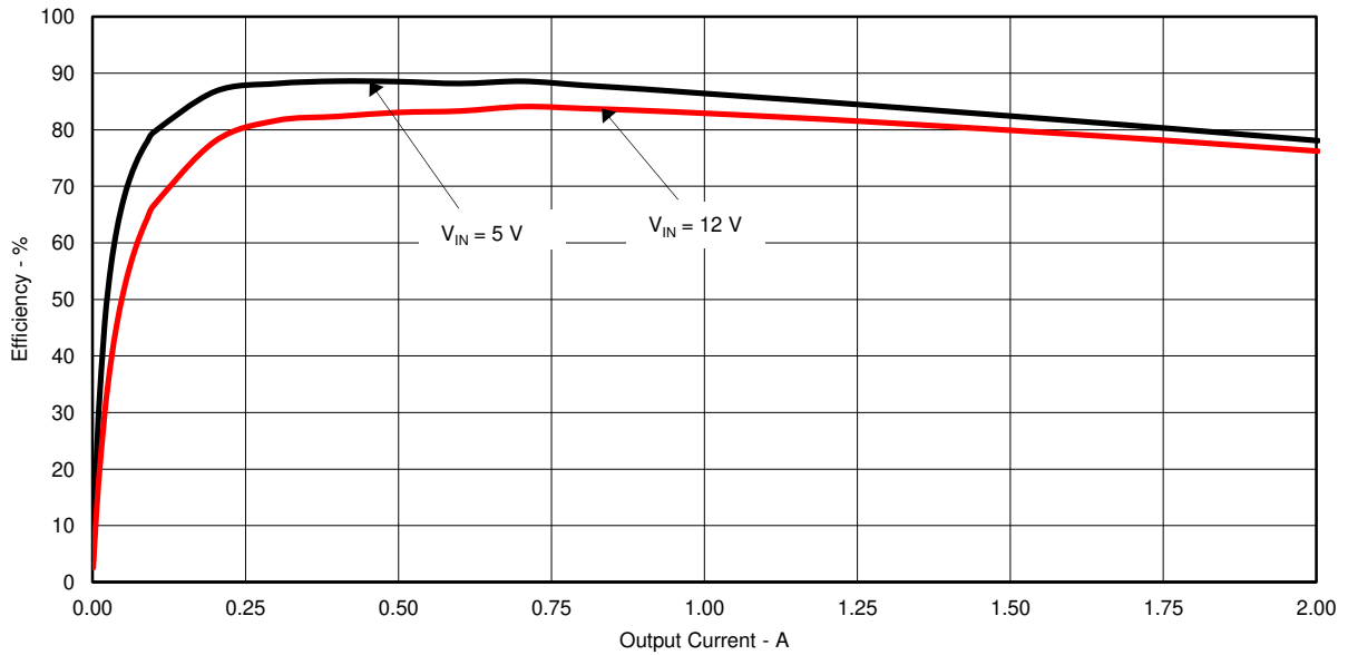
图 4-1. TPS562209EVM-601 效率
