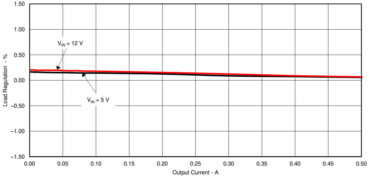
图 4-3. TPS562209EVM-601 负载调整率
