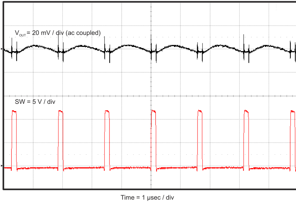
图 4-6. TPS562209EVM-601 输出电压纹波， I_{OUT} = 2A
