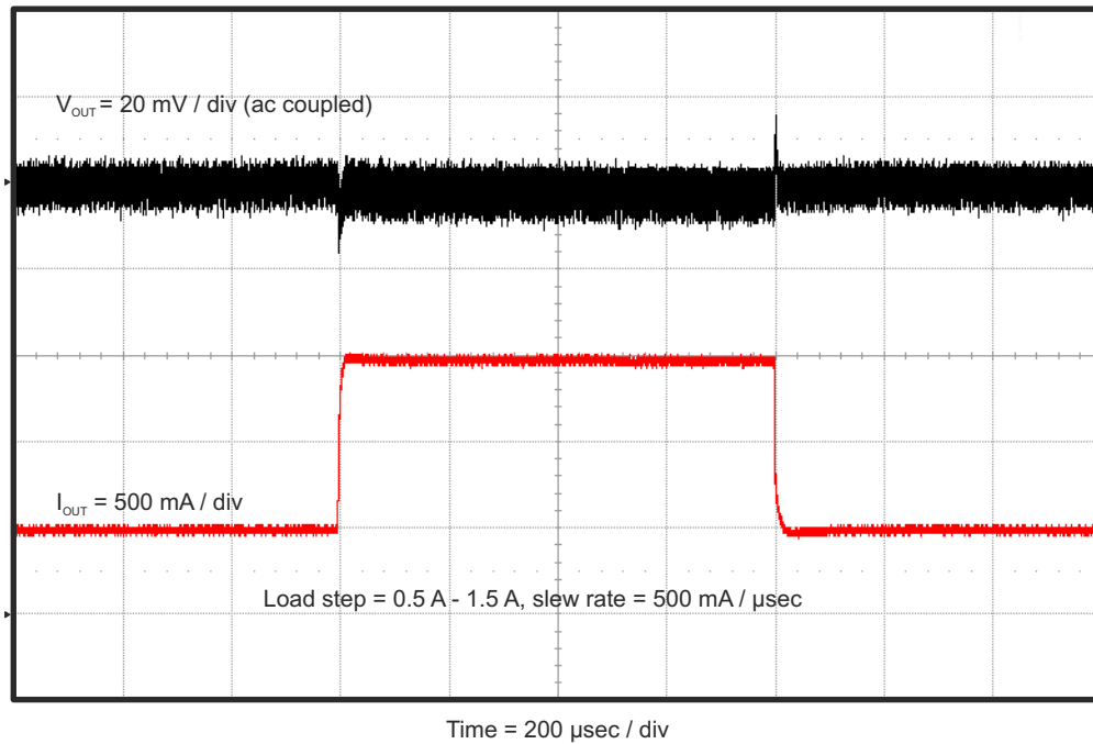
图 4-5. TPS562209EVM-601 负载瞬态响应，25% 至 75% 负载阶跃
