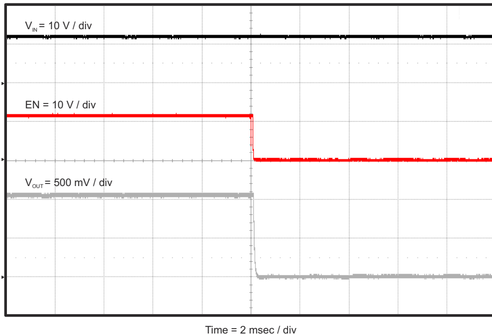
图 4-11. TPS562209EVM-601 相对于 EN 的关断波形
