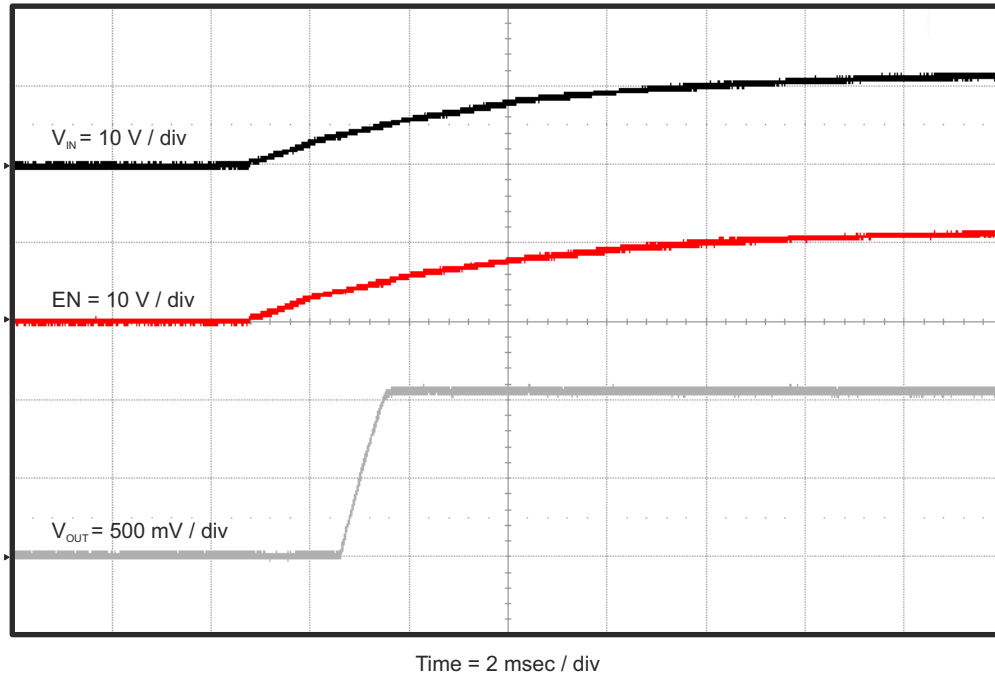
图 4-8. TPS562209EVM-601 相对于 V_{IN} 的启动波形
