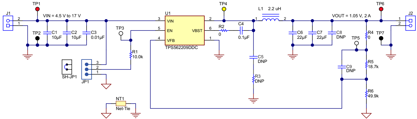
图 6-1. TPS562209EVM-601 原理图
