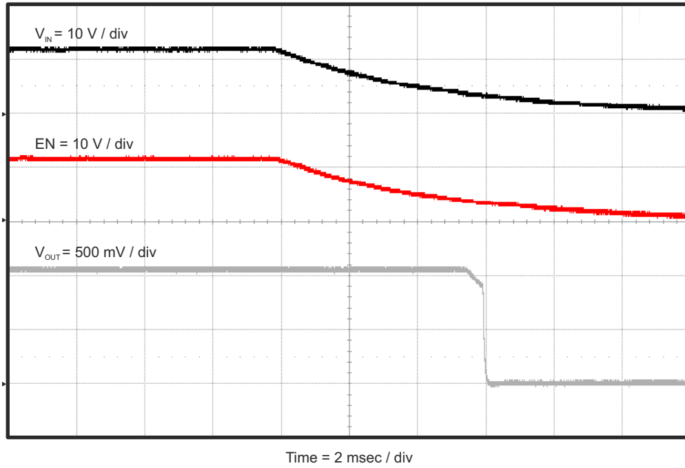
图 4-10. TPS562209EVM-601 相对于 V_{IN} 的关断波形
