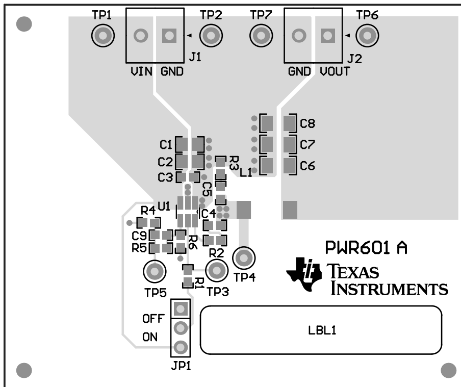
图 5-1. 顶层装配图
