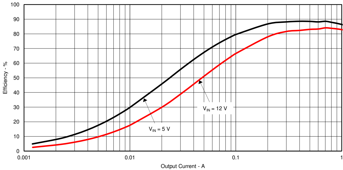
图 4-2. TPS562209EVM-601 轻负载效率
