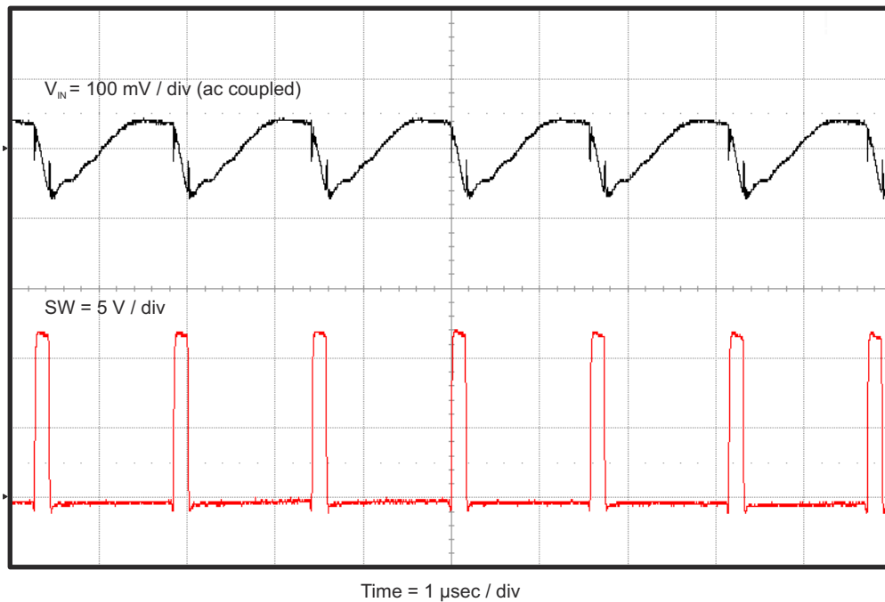
图 4-7. TPS562209EVM-601 输入电压纹波， I_{OUT} = 2A
