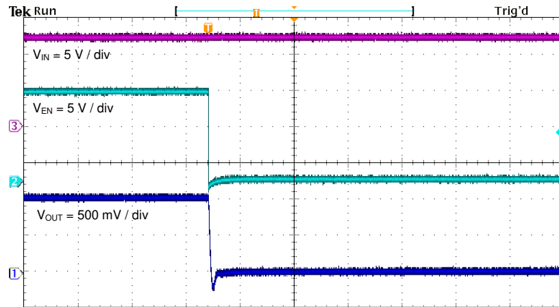
图 4-13. 相对于 EN 的关断
