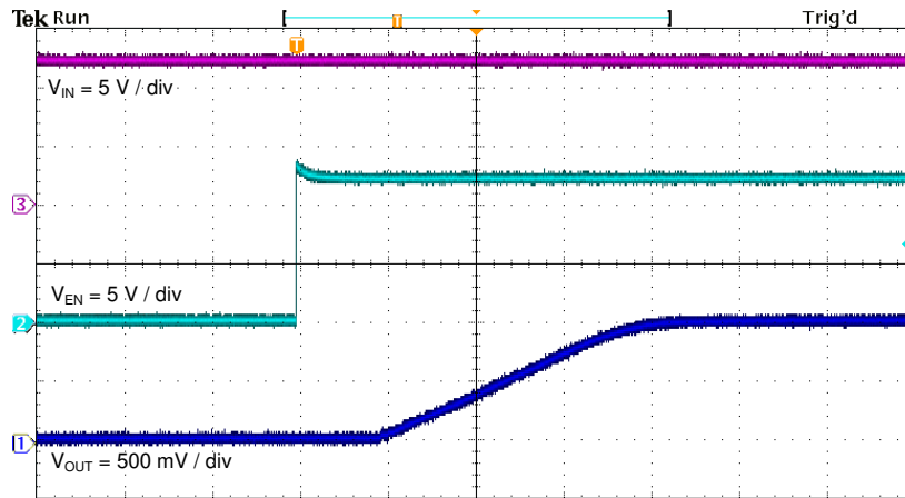
图 4-11. 相对于 EN 的启动
