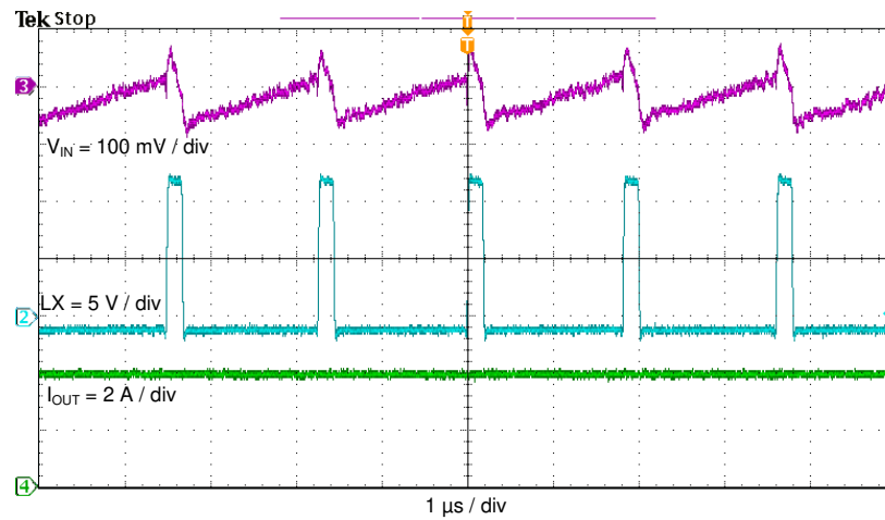
图 4-9. 输入电压纹波
