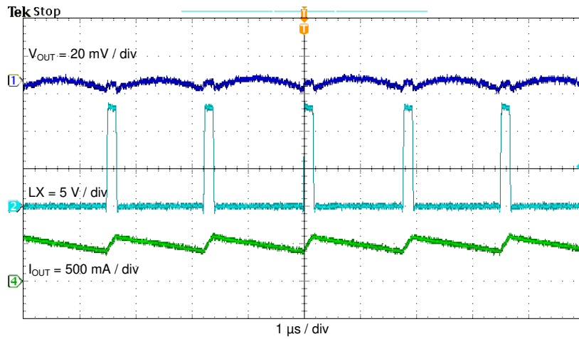
图 4-7. 输出电压纹波, I_{OUT} = 2\text{ A}
