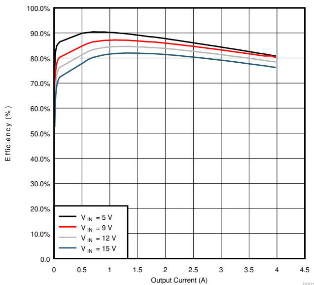
图 4-1. 效率
