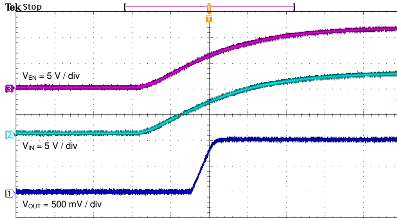
图 4-10. 相对于 V_{IN} 的启动
