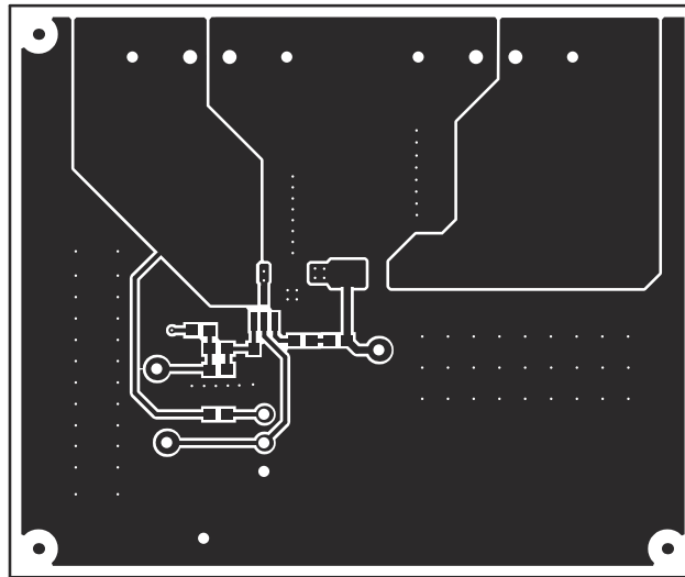
图 5-2. 顶层
