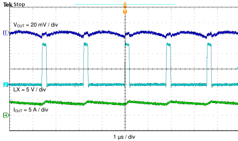
图 4-6. 输出电压纹波, I_{OUT} = 4\text{ A}
