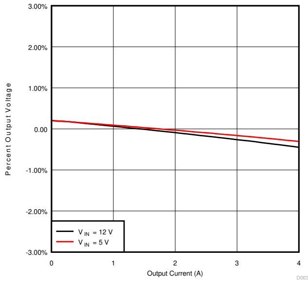
图 4-3. 负载调整率
