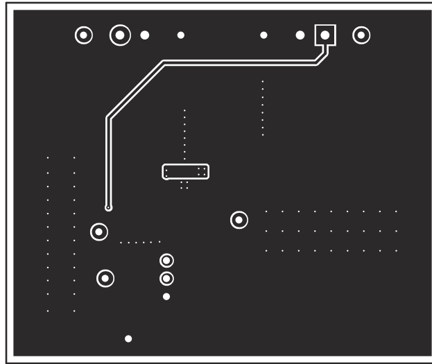
图 5-3. 底层
