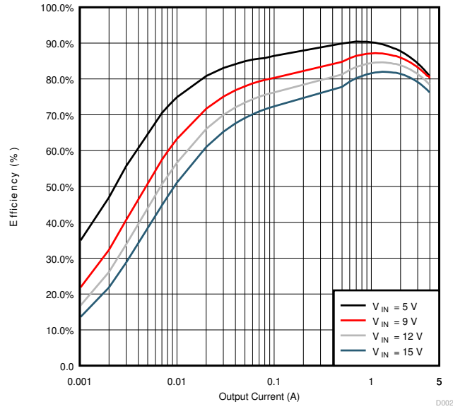
图 4-2. 轻负载效率
