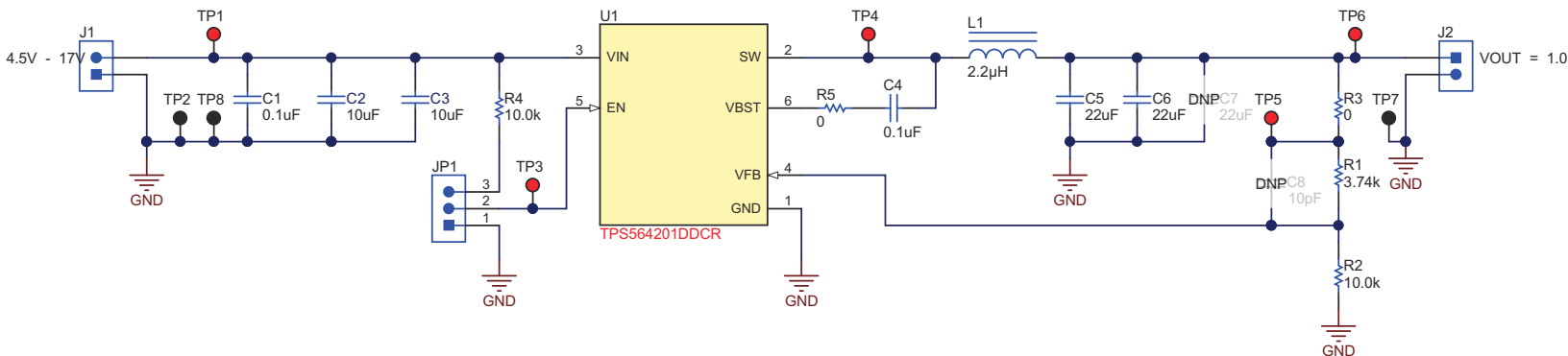
图 6-1. TPS564201EVM-801 原理图
