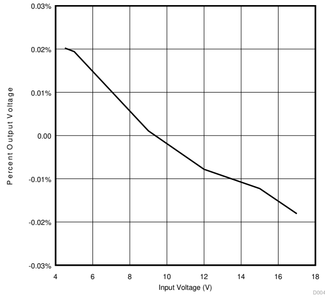
图 4-4. 线性调整率
