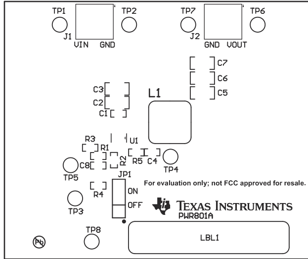
图 5-1. 顶层装配图
