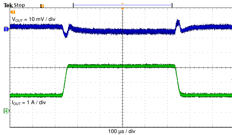
图 4-5. 负载瞬态响应，1 A 至 3 A
