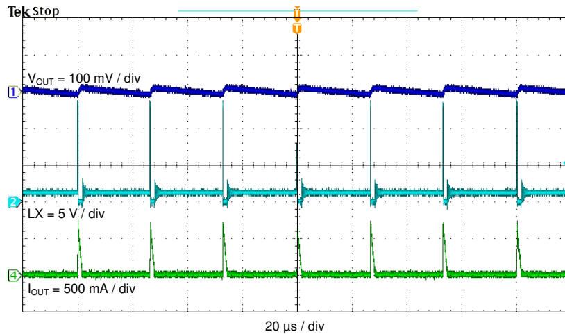
图 4-8. TPS564201 输出电压纹波, 无负载
