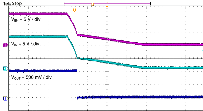
图 4-12. 相对于 V_{IN} 的关断
