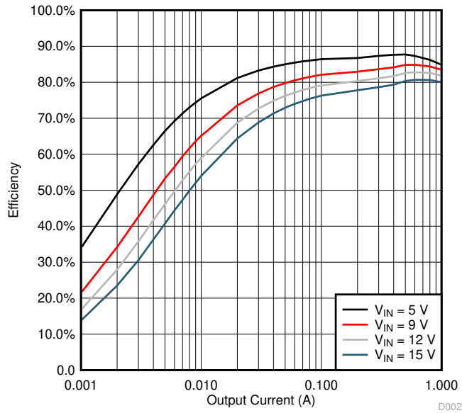
图 4-2. 轻负载效率
