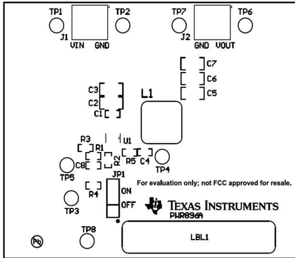
图 5-1. 顶层装配图
