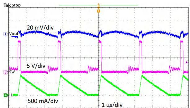
图 4-7. 输出电压纹波， I_{OUT} = 250\text{ mA}
