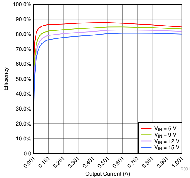
图 4-1. 效率
