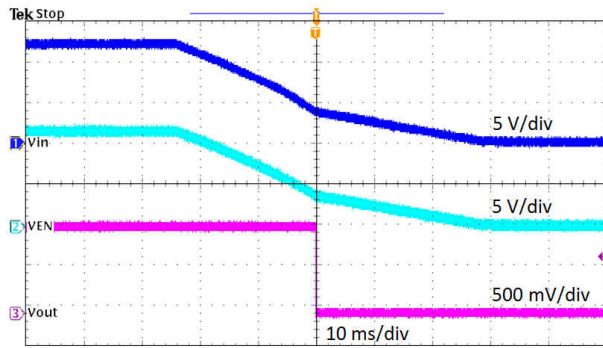
图 4-12. 相对于输入电压的关断
