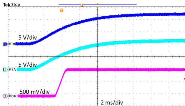
图 4-10. 相对于输入电压的启动
