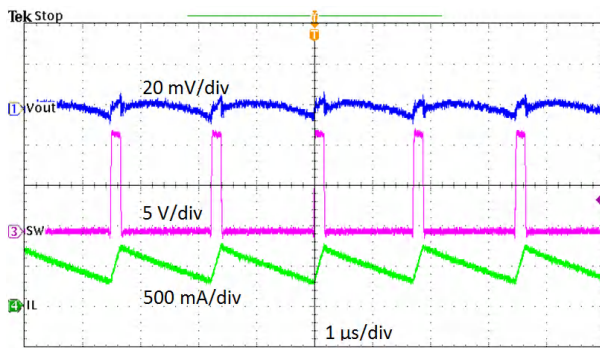
图 4-6. 输出电压纹波， I_{OUT} = 1\text{ A}
