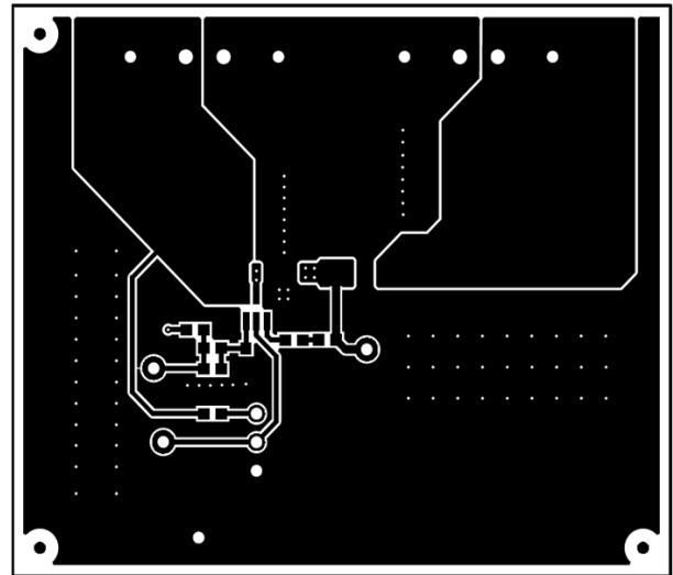
图 5-2. 顶层
