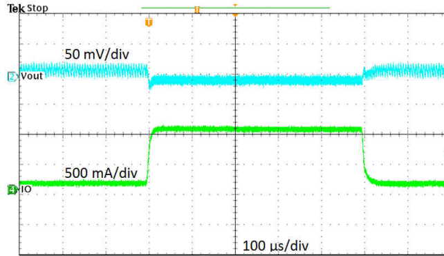
图 4-5. 负载瞬态响应，10% 至 100% 负载阶跃
