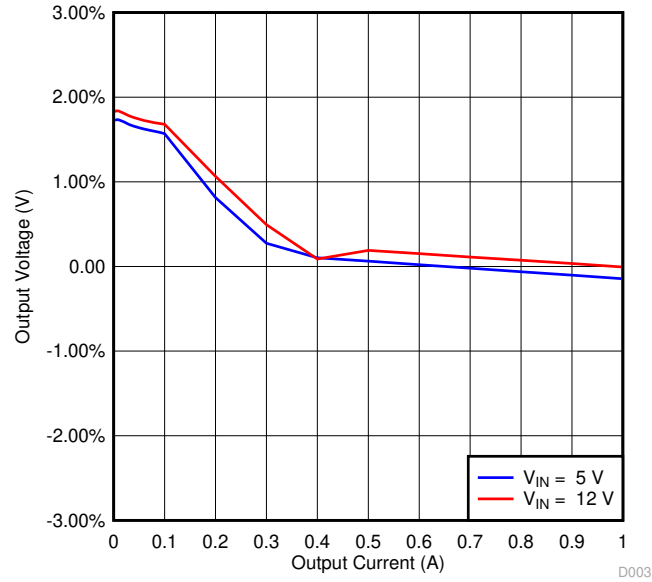
图 4-3. 负载调整率
