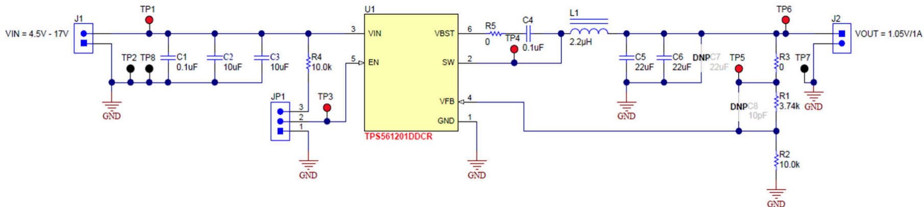
图 6-1. TPS561201EVM-896 原理图
