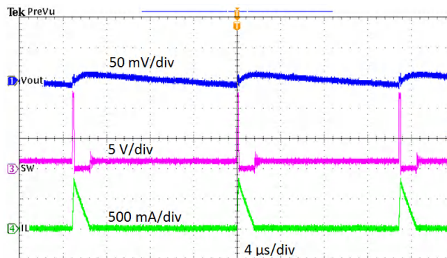
图 4-8. 输出电压纹波， I_{OUT} = 10\text{ mA}
