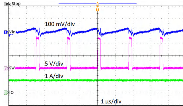
图 4-9. 输入电压纹波, I_{OUT} = 1 \text{ A}
