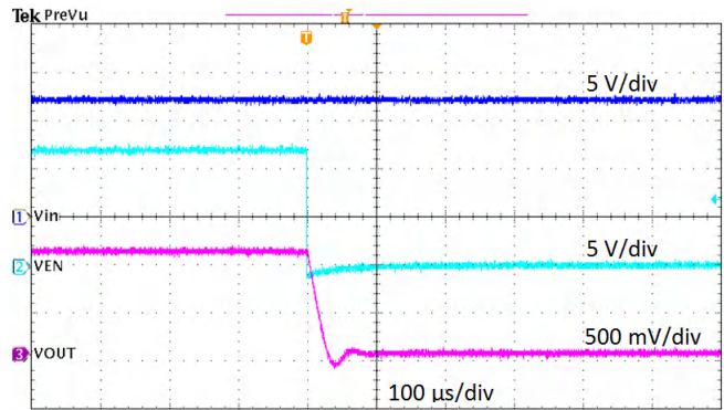
图 4-13. 相对于 EN 的关断
