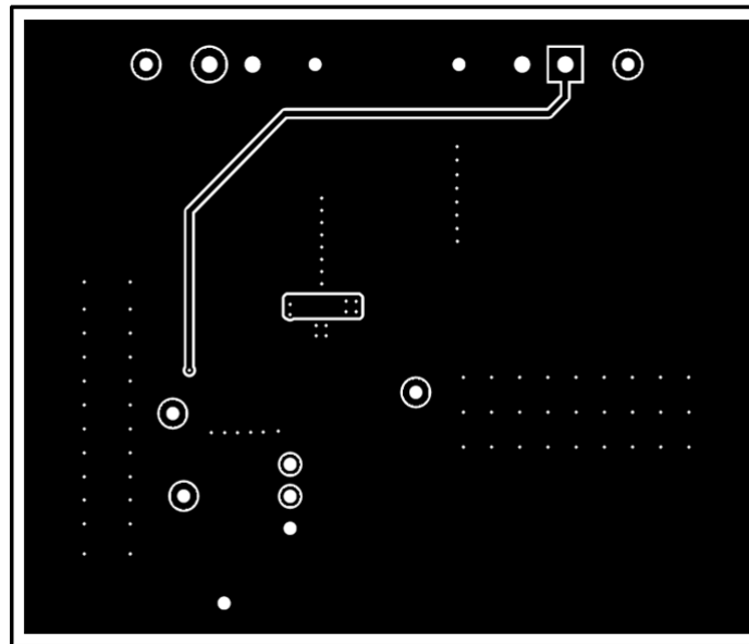
图 5-3. 底层
