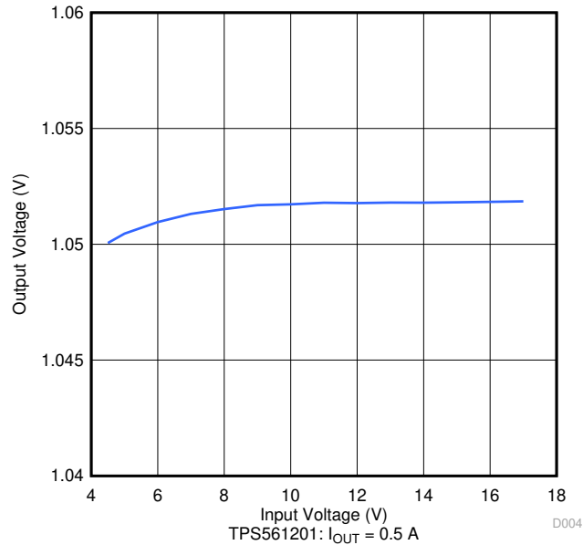
图 4-4. 线性调整率
