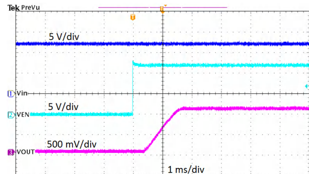
图 4-11. 相对于 EN 的启动
