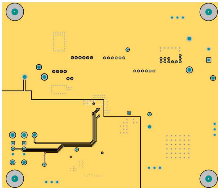
图 7-2. TPS923655DMTREV M 内层 1
