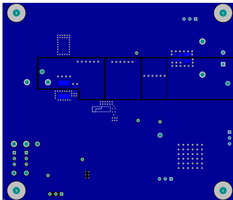
图 7-4. TPS923655DMTREV1 底层
