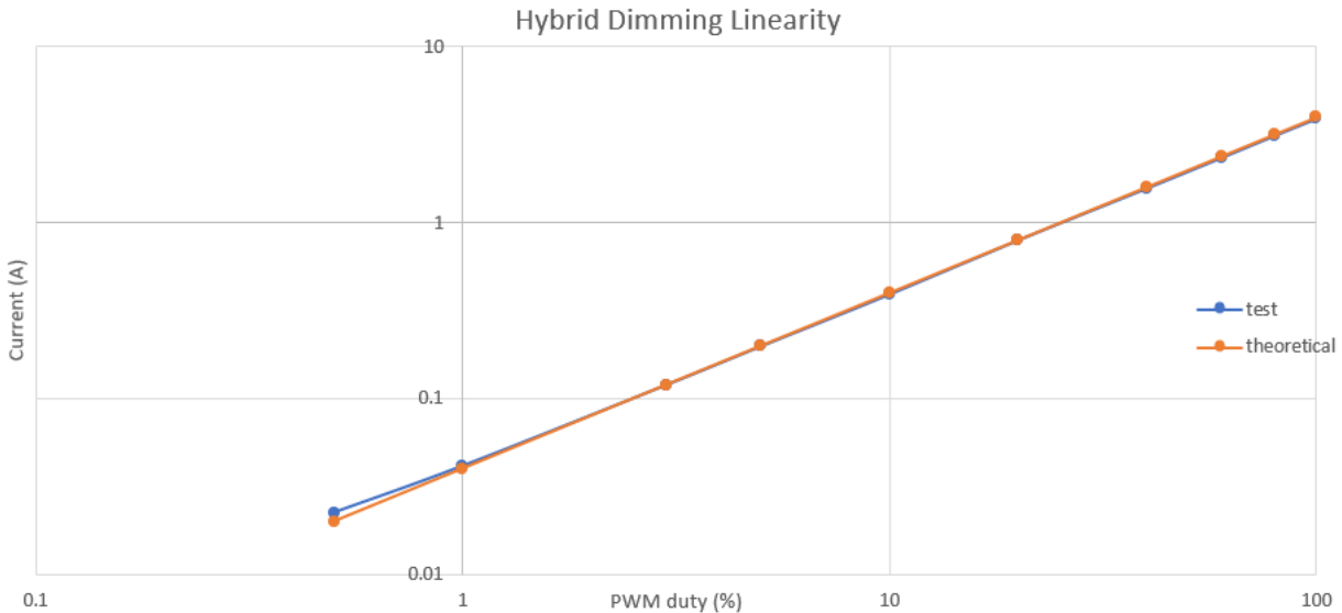
图 5-13. 混合调光线性
