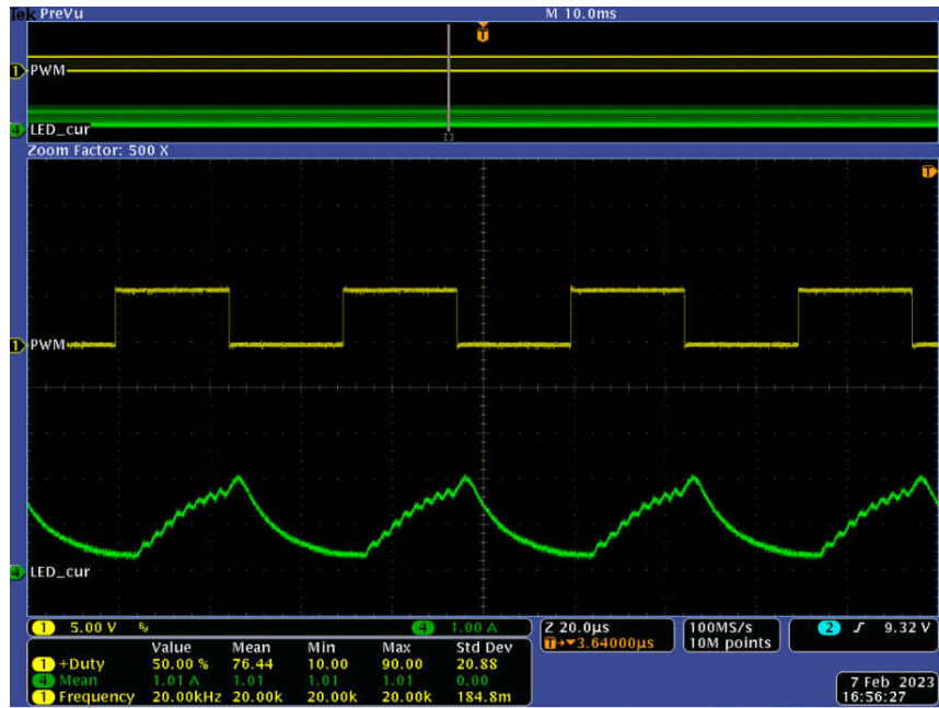
图 5-8. 50% 占空比、20kHz PWM 调光时的波形
