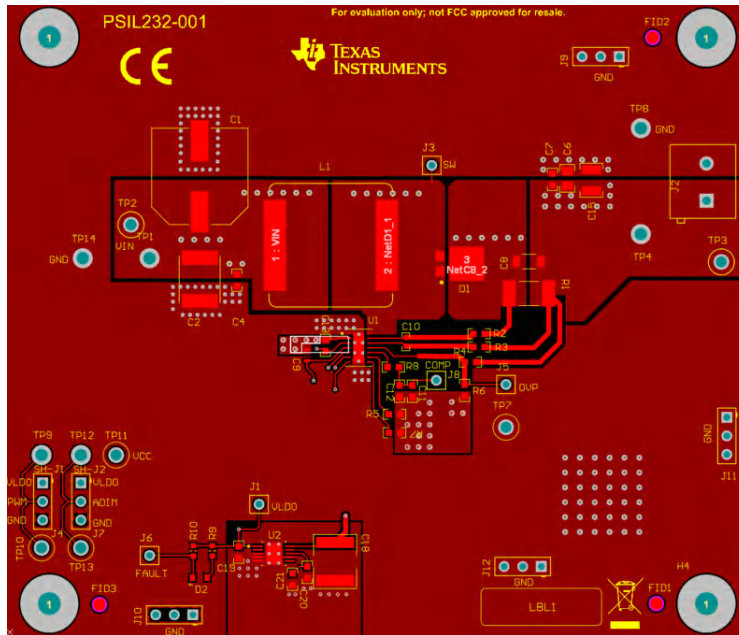
图 7-1. TPS923655DMTREV M 顶层
