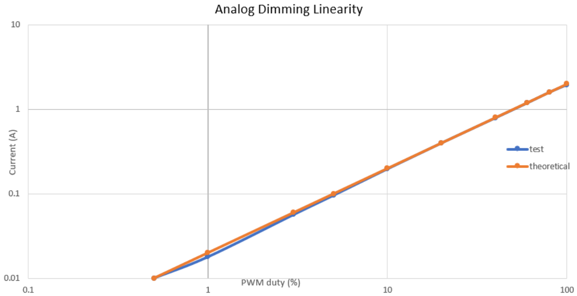
图 5-6. 模拟调光线性
