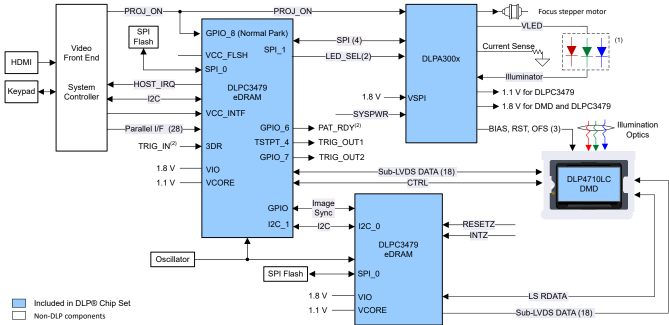
图 1-1. DLPC3479 系统方框图
