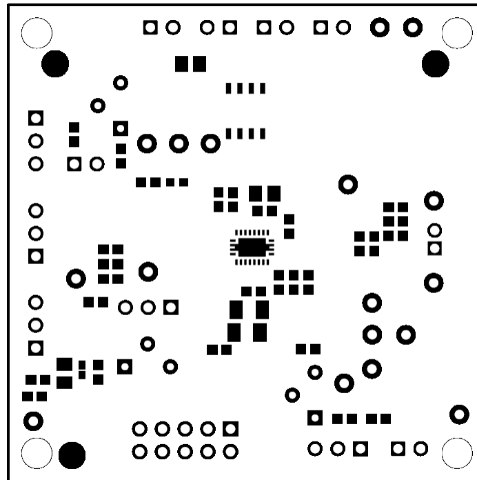
图 3-3. 顶部焊锡层
