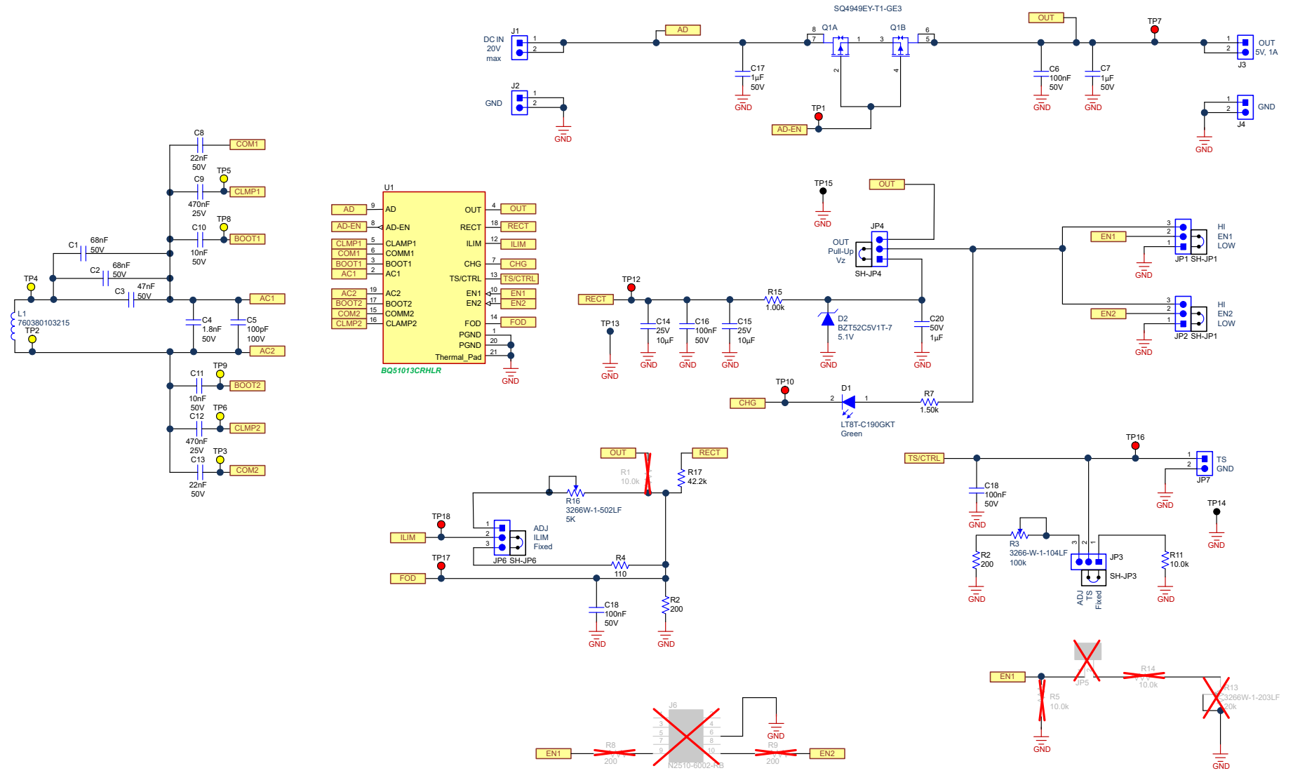
图 3-1. BQ51013C 原理图
