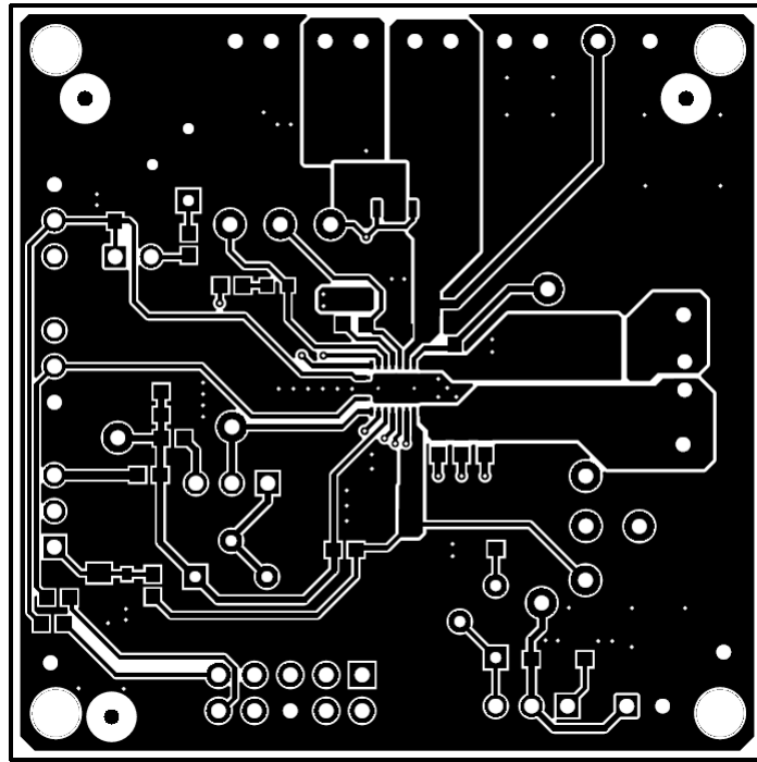
图 3-4. 顶层
