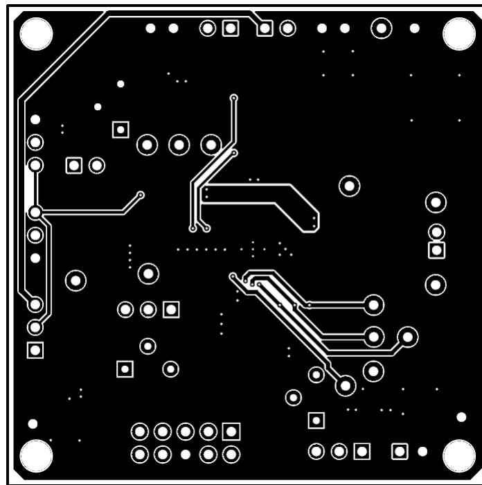
图 3-5. 底层
