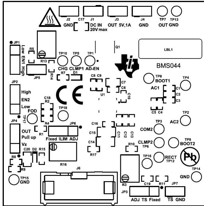
图 3-2. 顶层丝印层
