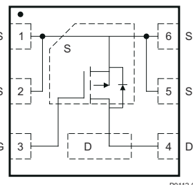
図 3-1. 上面図
