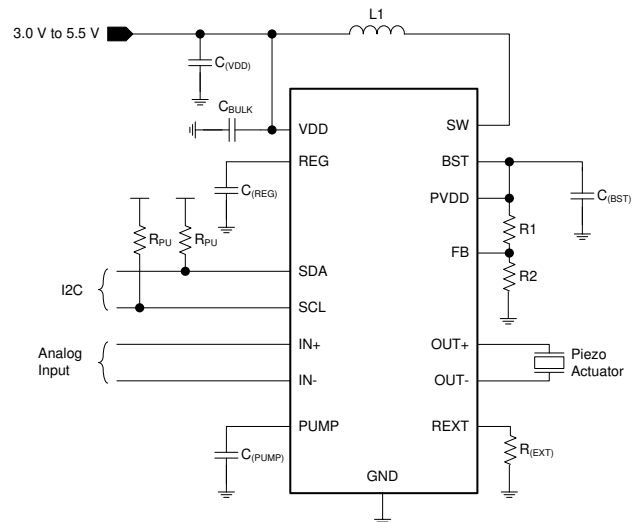
簡略回路図
