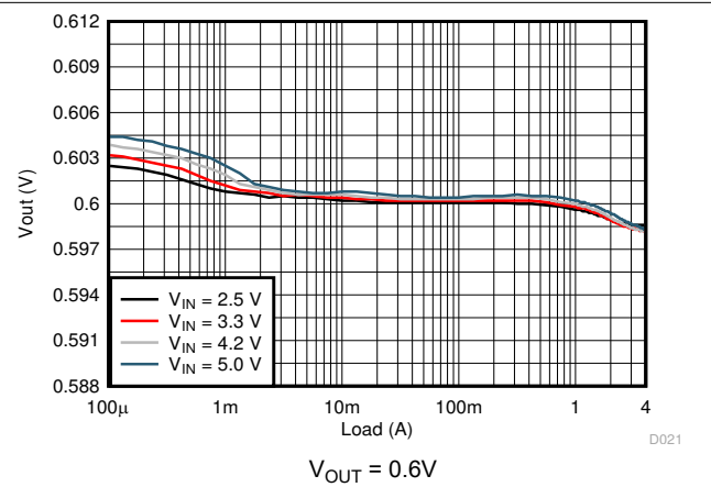
図 8-4. Load Regulation
