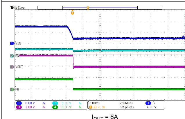
図 7-14. VIN Shutdown
