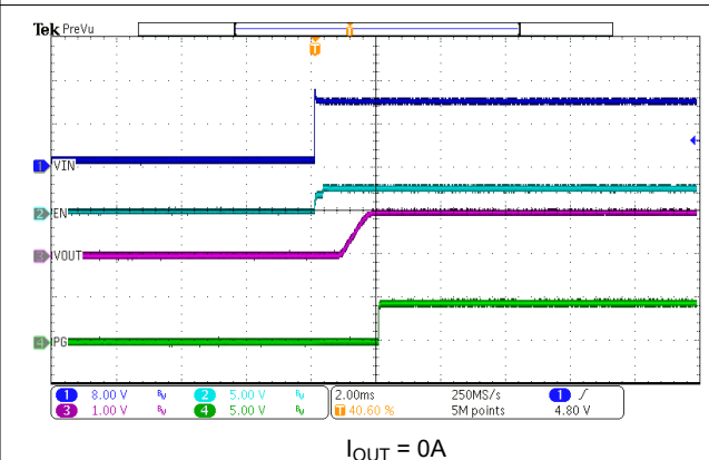
図 7-13. VIN Start-Up
