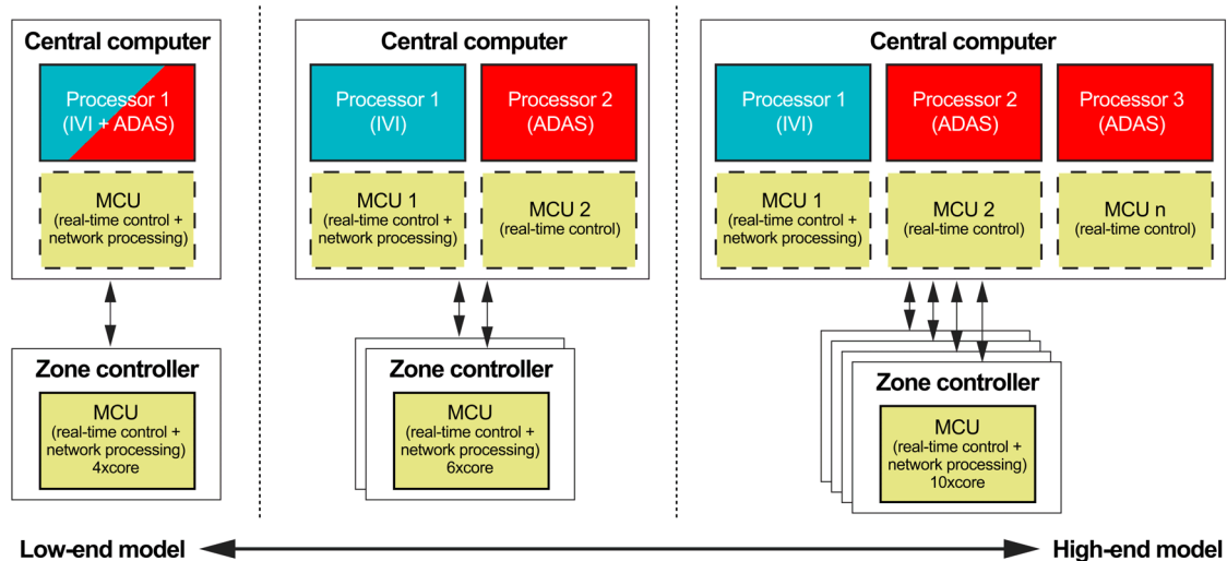
図3. ローエンドとハイエンドの車両モデル間の計算能力の比較。
