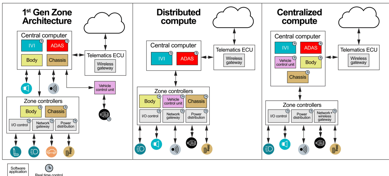
図5. 自動車アーキテクチャの種類の比較。
