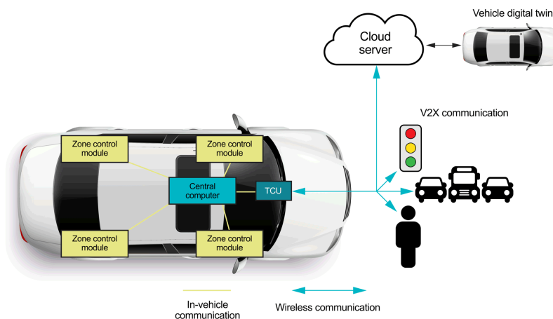
図4. クラウドと V2X へのソフトウェア定義自動車の接続性。
