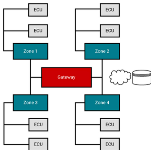
図 2. 自動車におけるゾーン アーキテクチャの図表。
